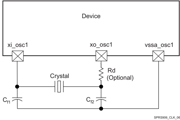
图 6-6. Crystal Implementation
