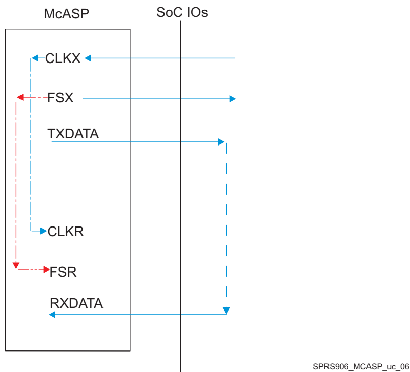
图 7-48. McASP1-8 CI-FO- - SYNC Mode
