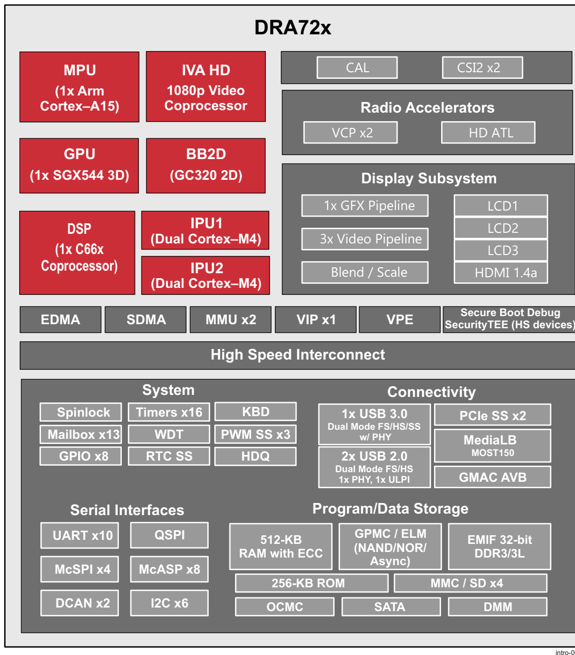
图 1-1. DRA72x 方框图
