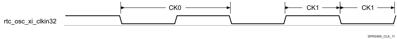
图 6-13. rtc_osc_xi_clkin32 Input Clock
