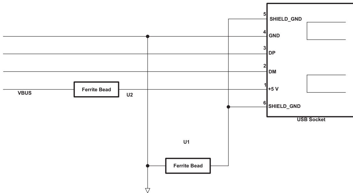
图 8-23. USB Connector
