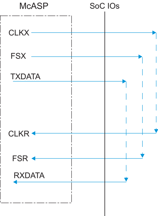
图 7-43. McASP1-8 COIFOI - ASYNC Mode
