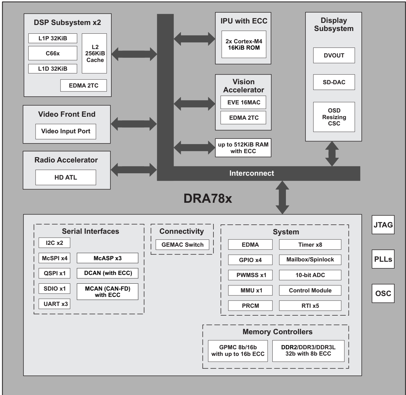
图 1-1. DRA78x 框图
