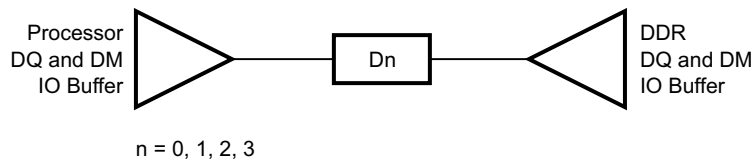
图 7-52. DQ/DM Topology
