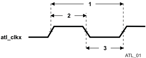
图 5-62. ATL_CLKOUTx Timing
