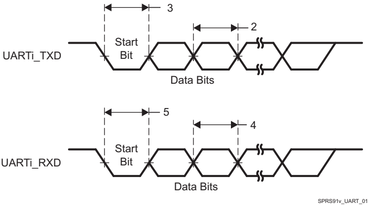
图 5-40. UART Timing
