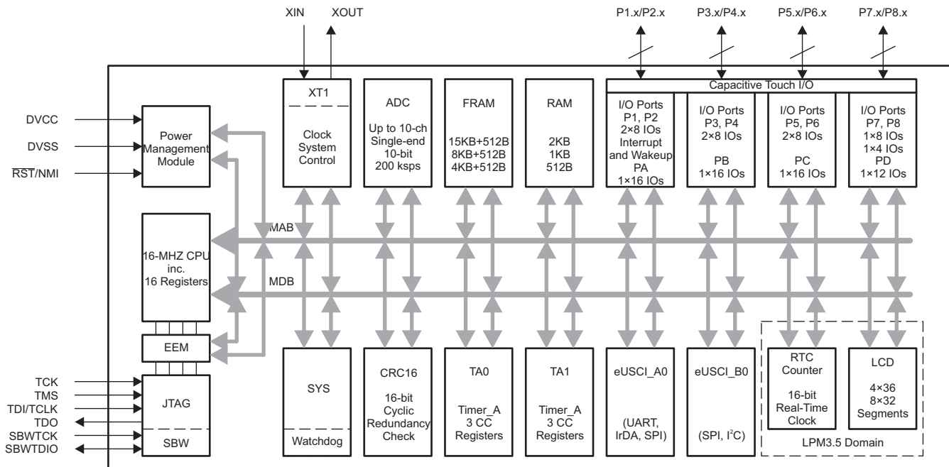
图 1-1. 功能框图
