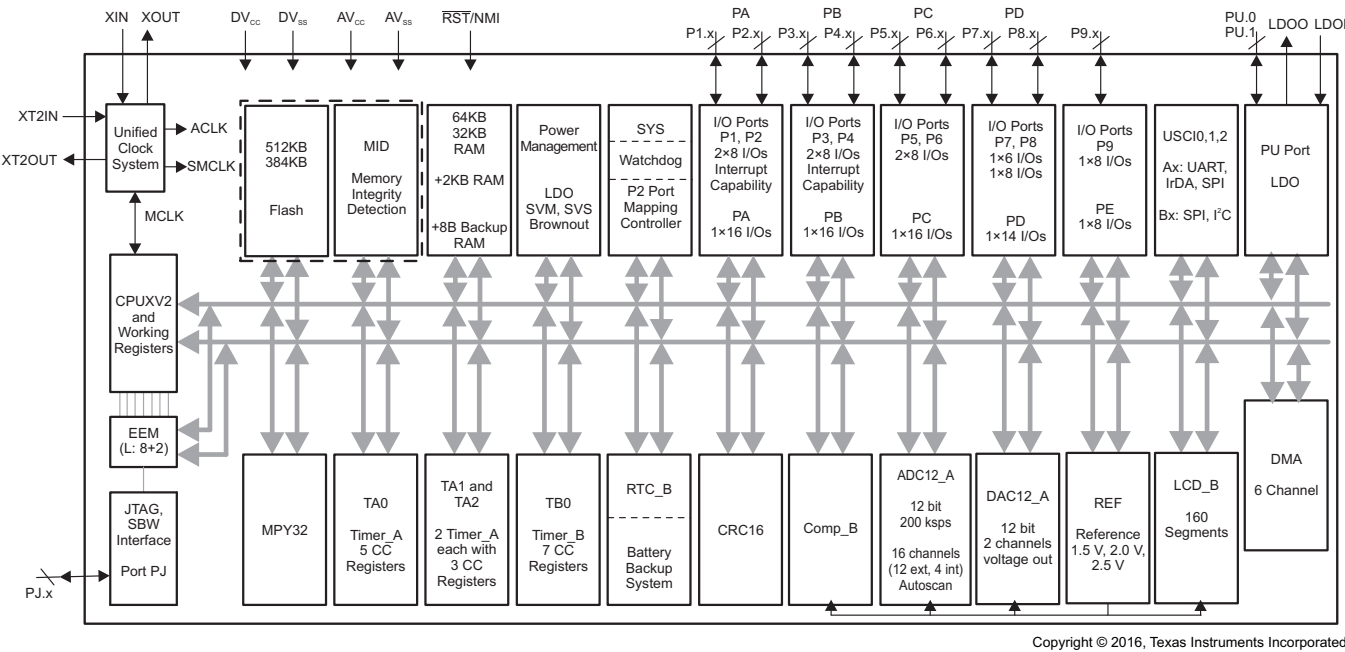
图 1-1. 功能方框图
