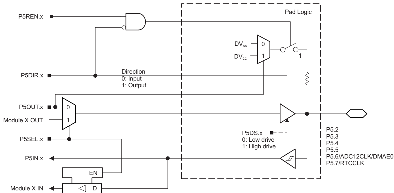
图 6-7. Port P5 (P5.2 to P5.7) Diagram
