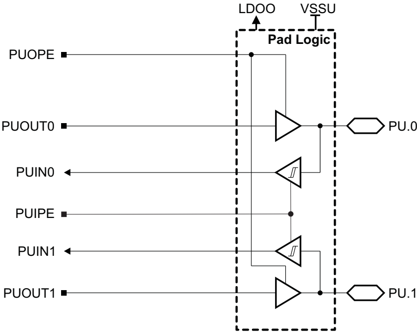
图 6-14. Port PU (PU.0 and PU.1) Diagram
