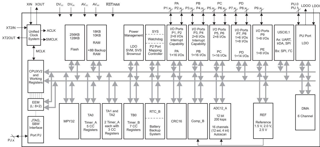
图 1-2. 功能框图 – MSP430F5335 和 MSP430F5333
