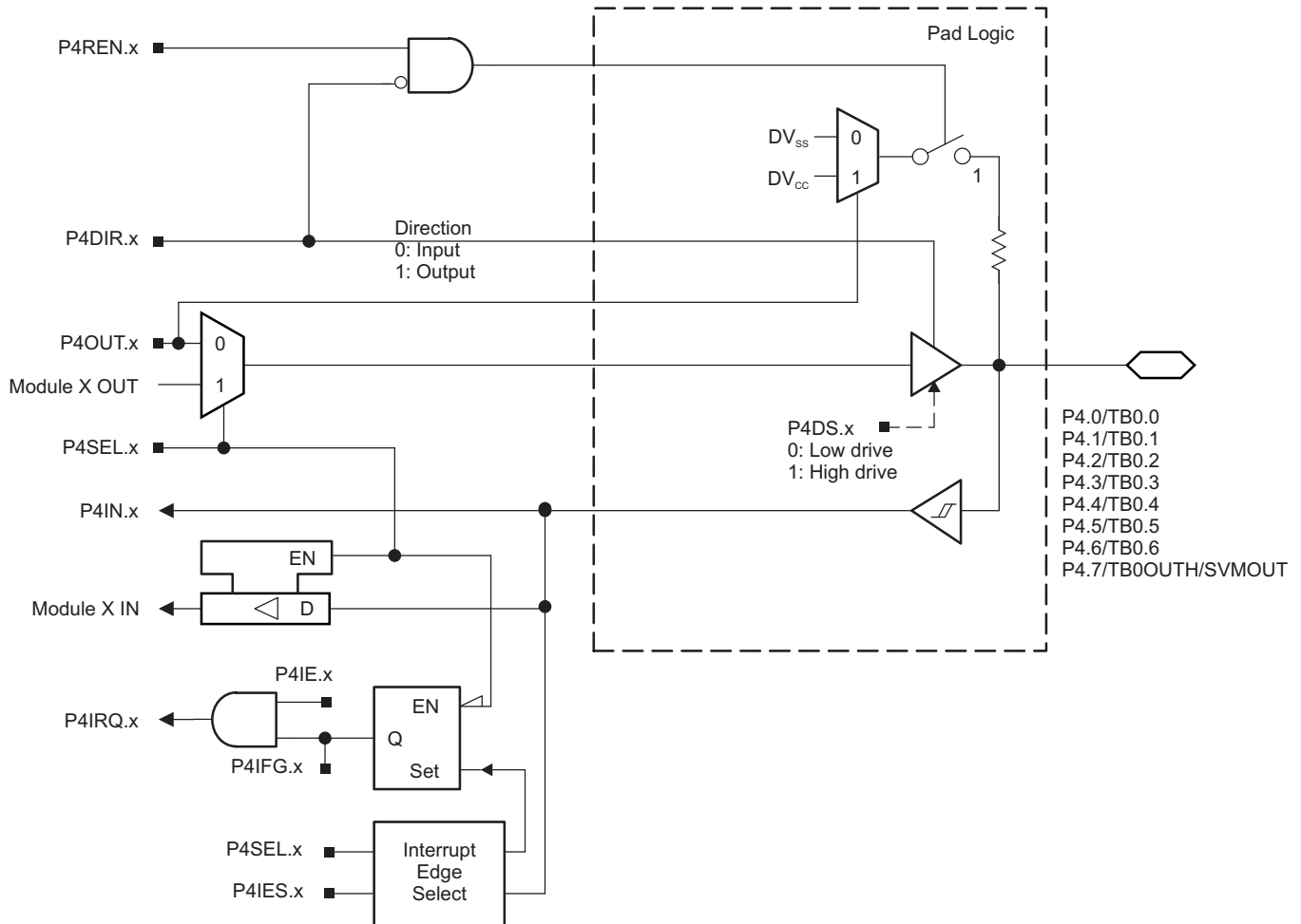
图 6-5. Port P4 (P4.0 to P4.7) Diagram
