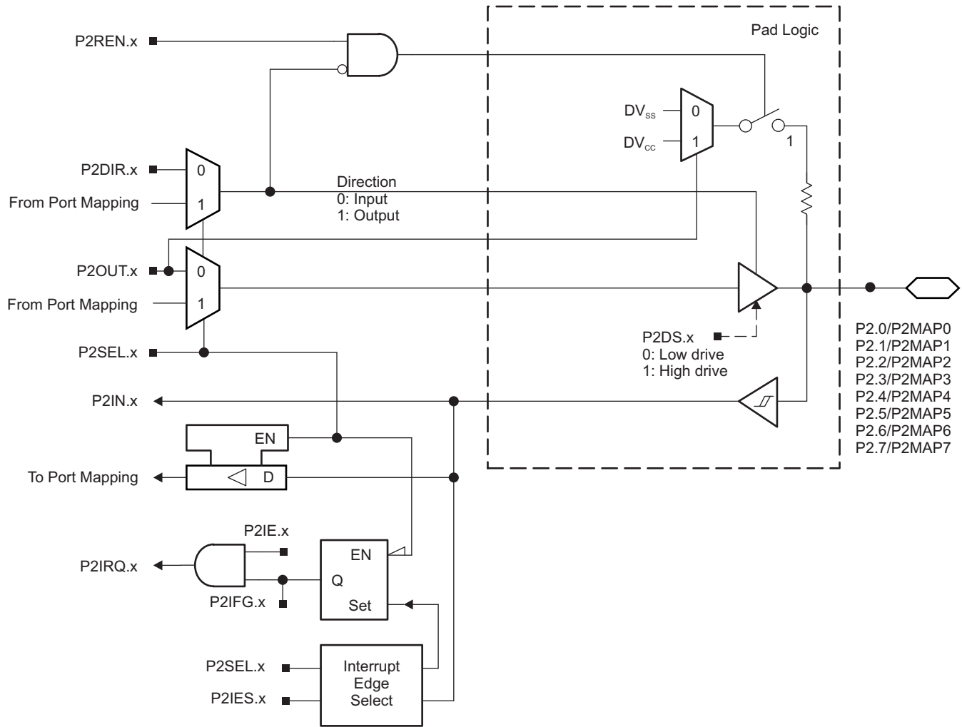
图 6-3. Port P2 (P2.0 to P2.7) Diagram
