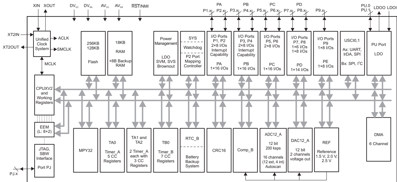
图 1-1. 功能框图 – MSP430F5338 和 MSP430F5336
