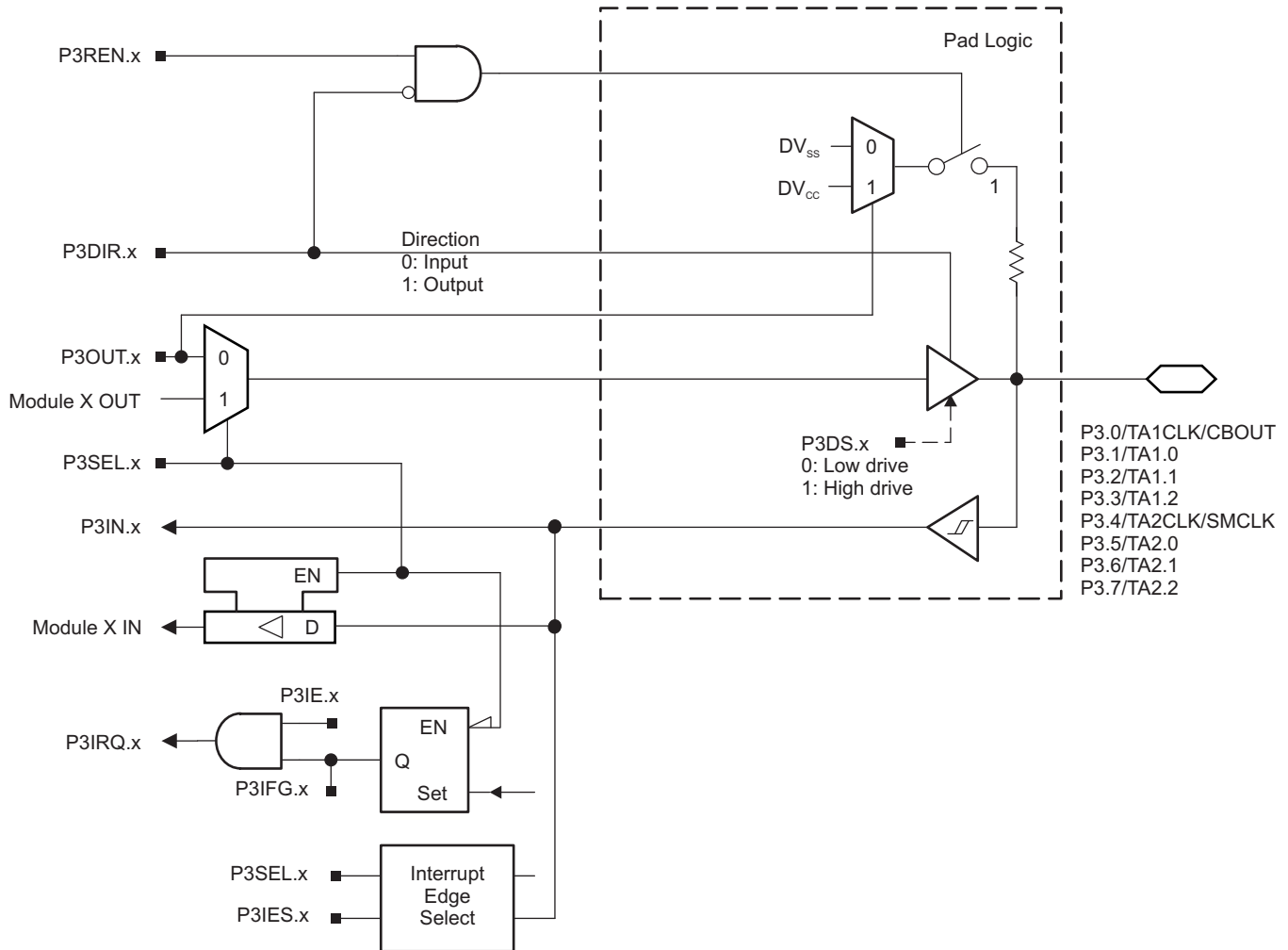
图 6-4. Port P3 (P3.0 to P3.7) Diagram
