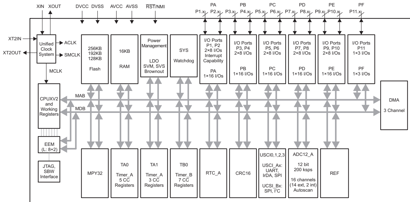
图 1-1. 功能方框图 - MSP430F5438AIPZ、MSP430F5436AIPZ、MSP430F5419AIPZ、MSP430F5438AIZQW、MSP430F5436AIZQW、MSP430F5419AIZQW
