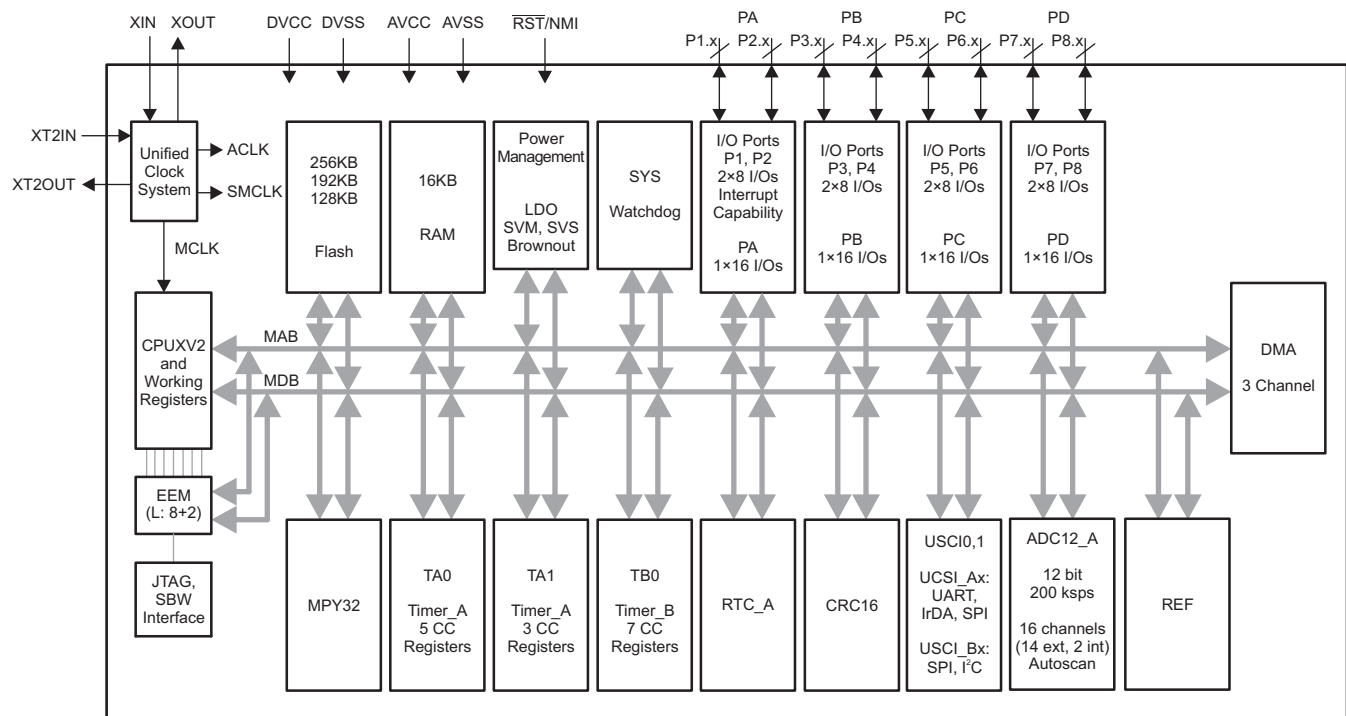
图 1-2. 功能方框图 - MSP430F5437AIPN、MSP430F5435AIPN、MSP430F5418AIPN
