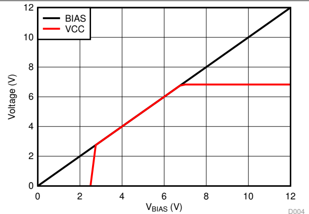
图 4. VCC vs V_BIAS (No Load)
