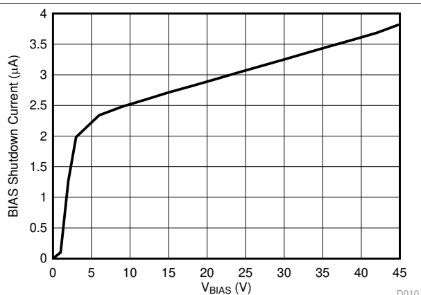
图 10. I_{\text{SHUTDOWN}}(\text{BIAS}) vs V_{\text{BIAS}}
