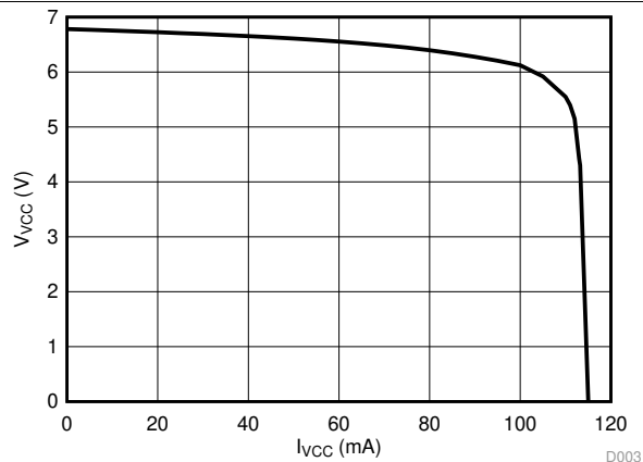
图 3. VCC vs I_VCC
