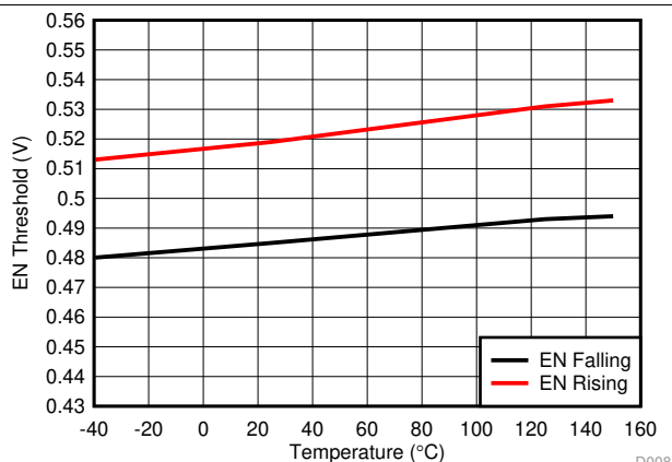
图 8. EN Threshold vs Temperature
