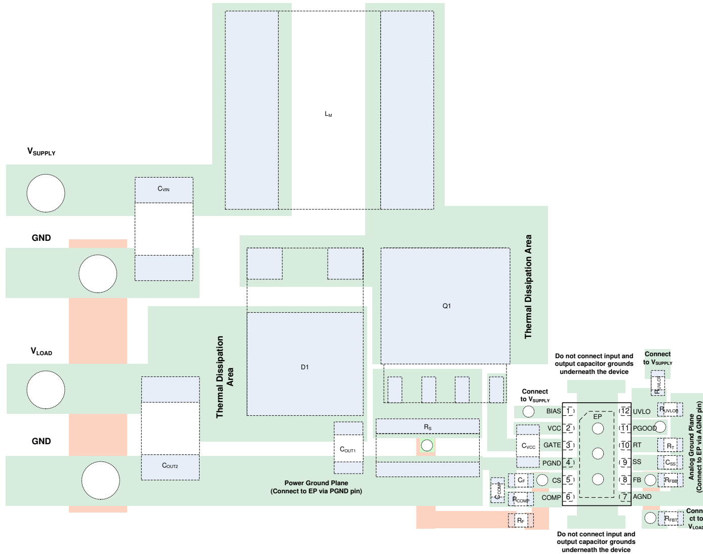
图 52. PCB Layout Example 2
