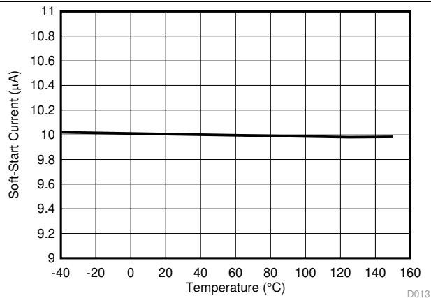
图 13. I_{SS} vs Temperature
