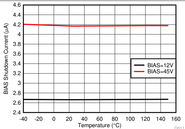
图 11. I_{\text{SHUTDOWN}} vs Temperature
