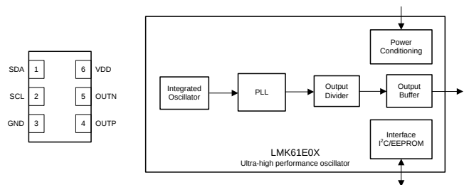
引脚分布和简化框图
