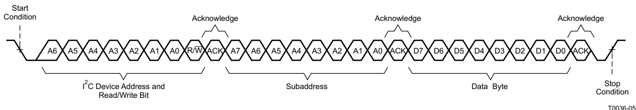
图 14. Random Write Transfer
