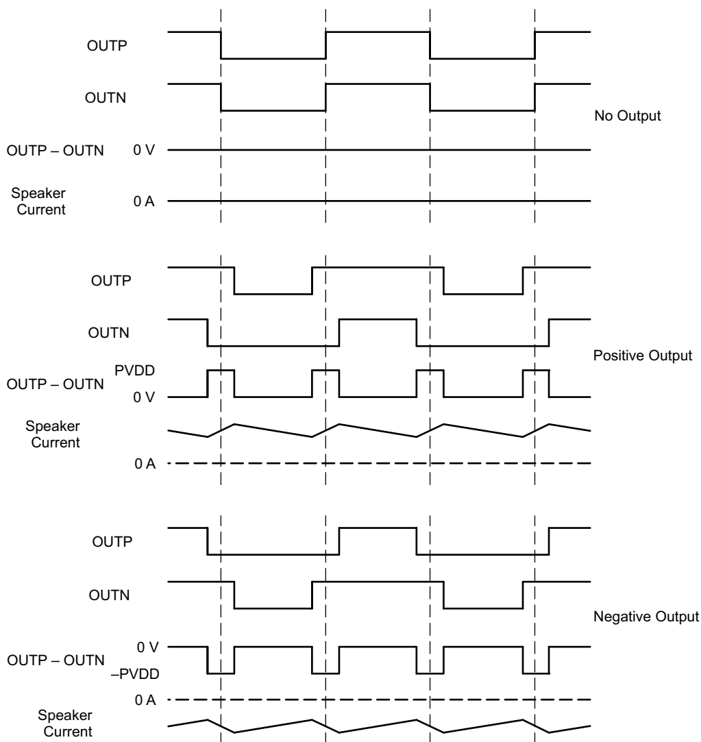
图 10. BD Mode Modulation
