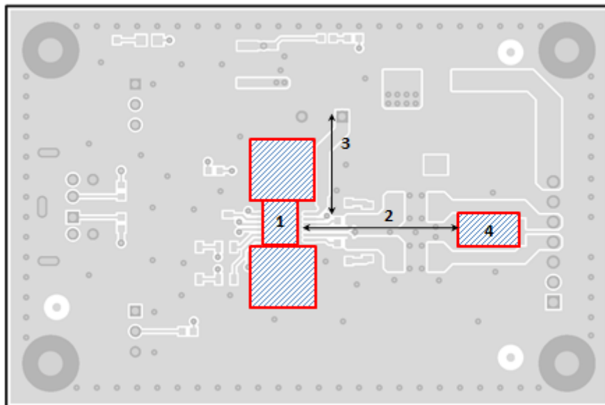
图 18. Top Layer
