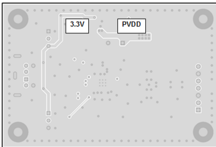
图 20. Power Layer
