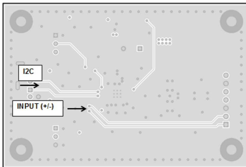
图 19. Signal Layer
