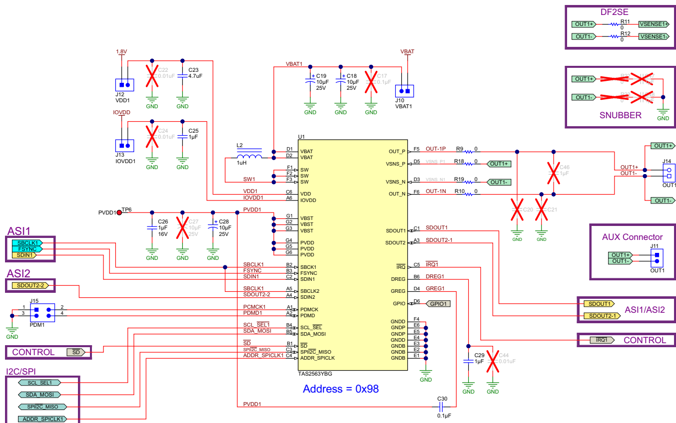
图 48. TAS2563 Circuit
