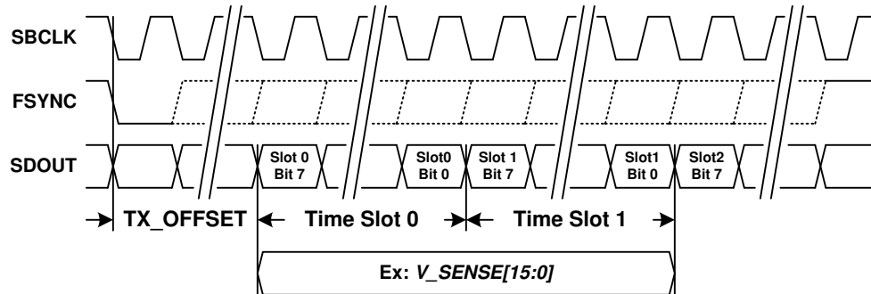
图 61. TDM Port TX Diagram
