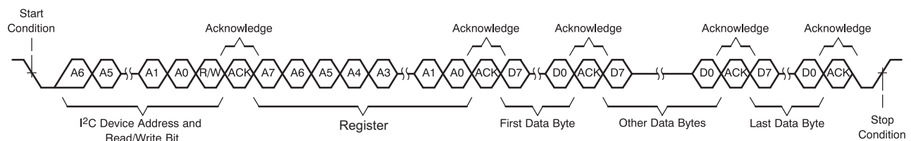
图 54. Multi-Byte Write Transfer
