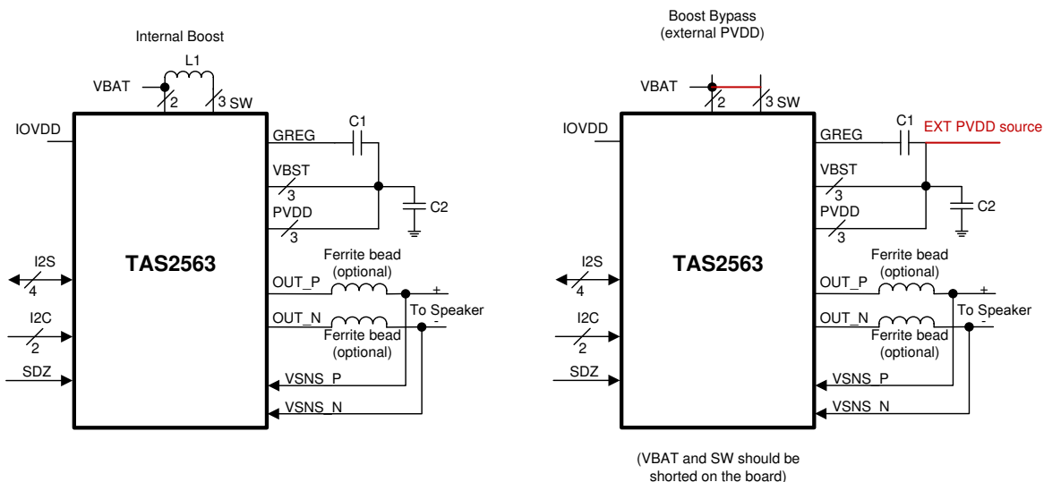
简化原理图
