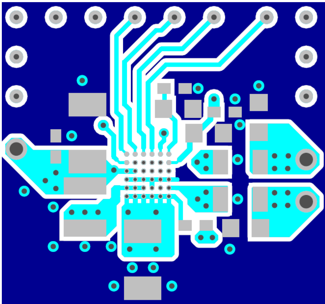
图 133. TAS2563 Top Copper Layout
