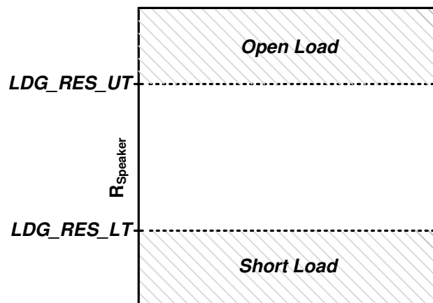
图 67. Load Diagnostics
