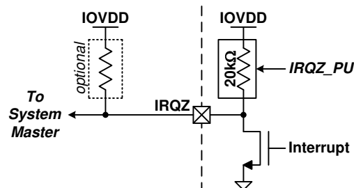
图 57. IRQZ Pin
