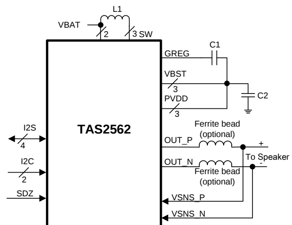
简化原理图
