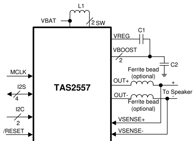
简化原理图
