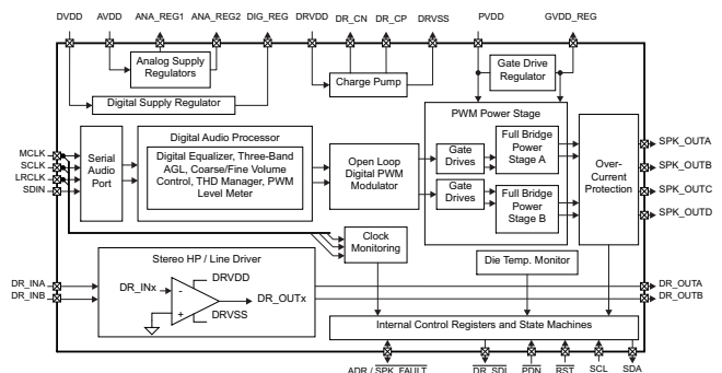
功能方框图
