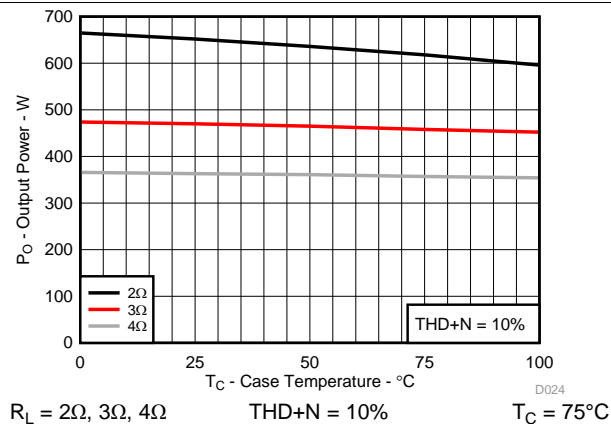
图 24. Output Power vs Case Temperature
