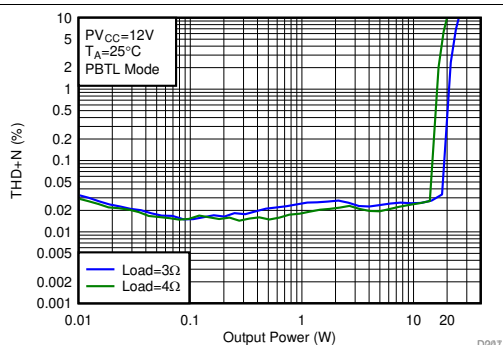
图 70. THD+N vs Output Power-PBTL
