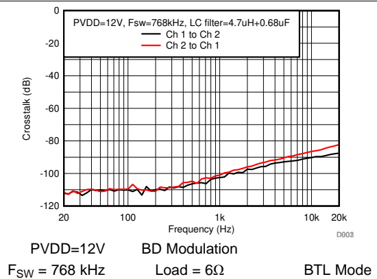
图 59. Crosstalk
