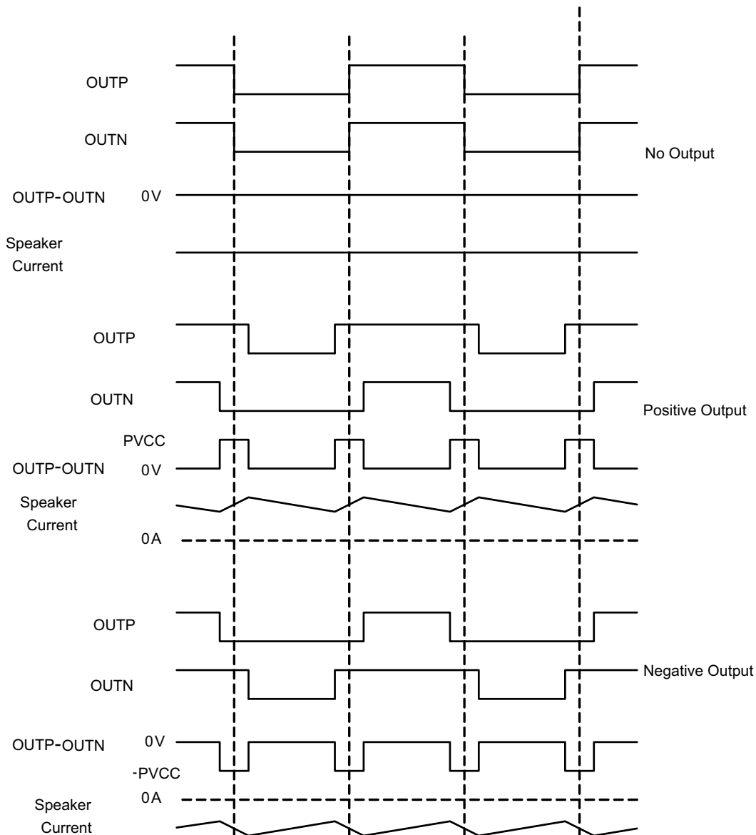
图 87. BD Mode Modulation
