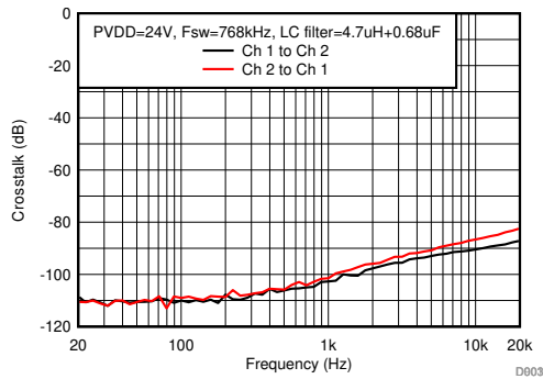
图 60. Crosstalk
