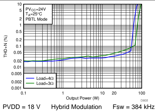
图 161. THD+N vs Output Power
