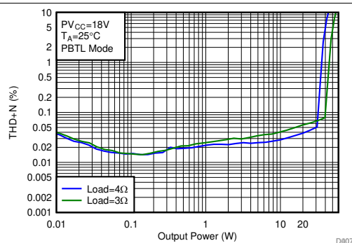
图 30. THD+N vs Output Power-PBTL
