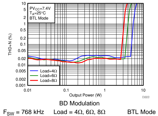
图 49. THD+N vs Output Power-BTL
