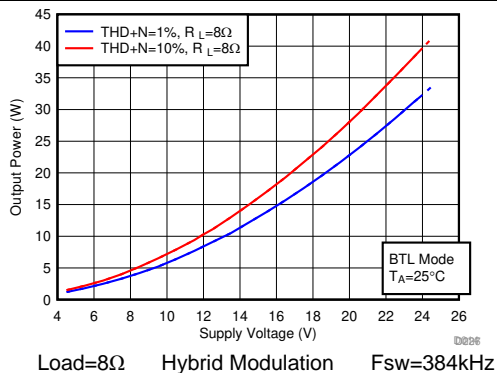
图 153. Output Power vs PVDD
