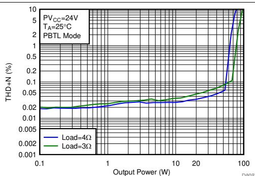
图 29. THD+N vs Output Power-PBTL
