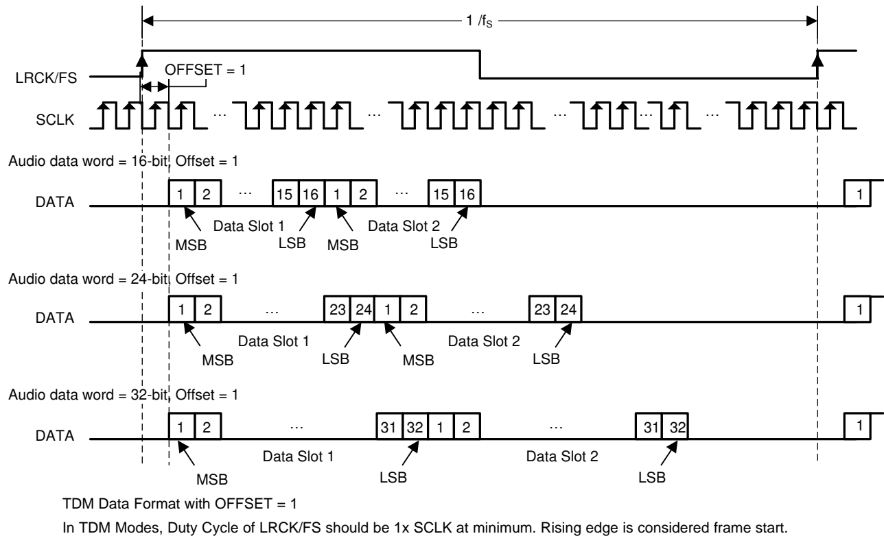
图 85. TDM 2 Audio Data Format
