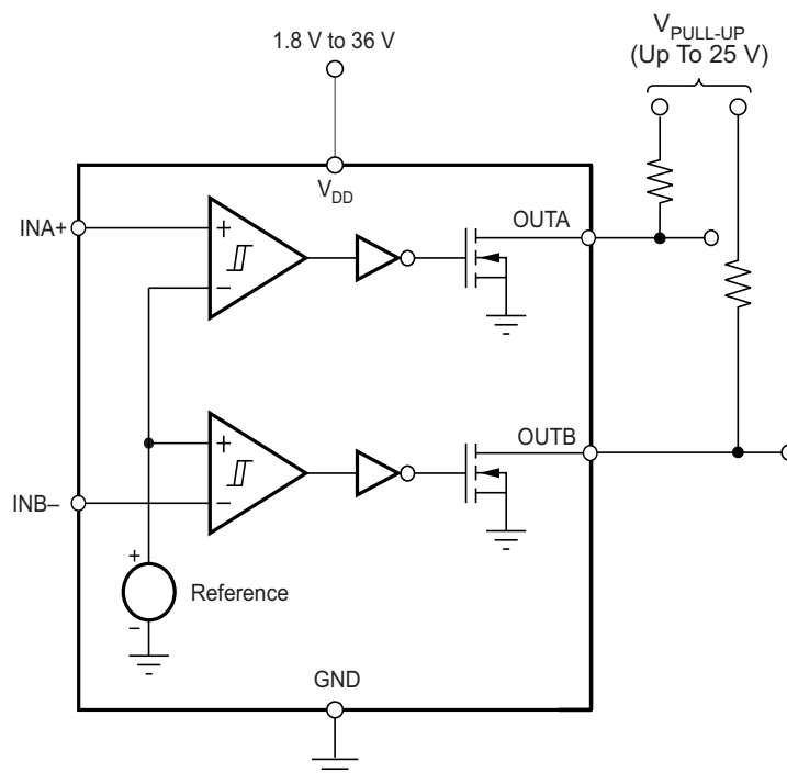
简化框图
