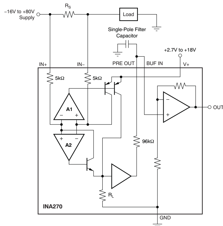
简化原理图
