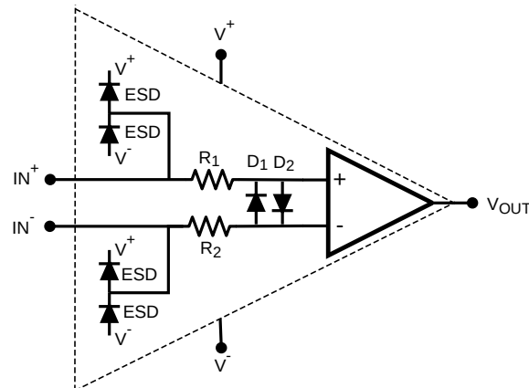
图 34. 输入引脚之间的保护二极管
