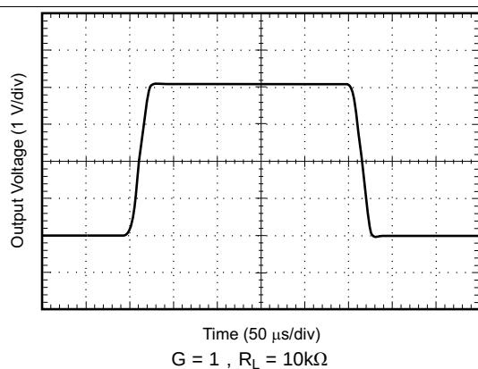
Figure 9. 大信号阶跃响应
