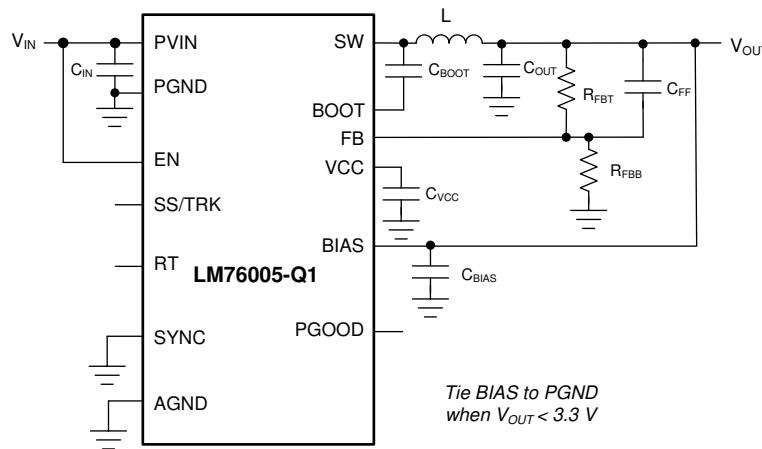
图 15. LM76005-Q1 Basic Schematic
