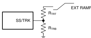
图 9. Soft-Start Tracking External Ramp
