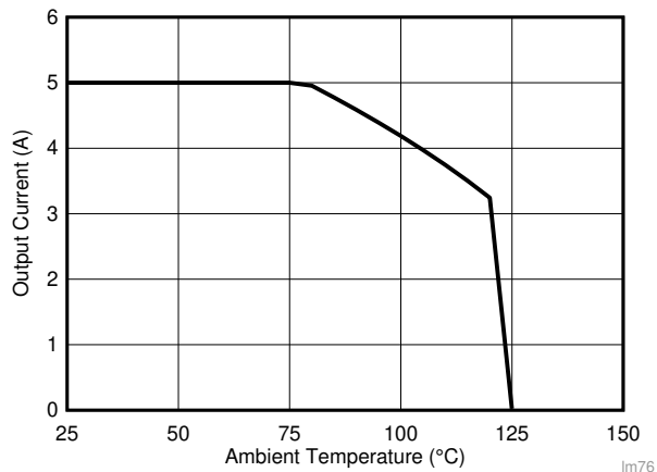
图 17. LM76005-Q1 Safe Operating Area (5 V OUT , 400 kHz)
