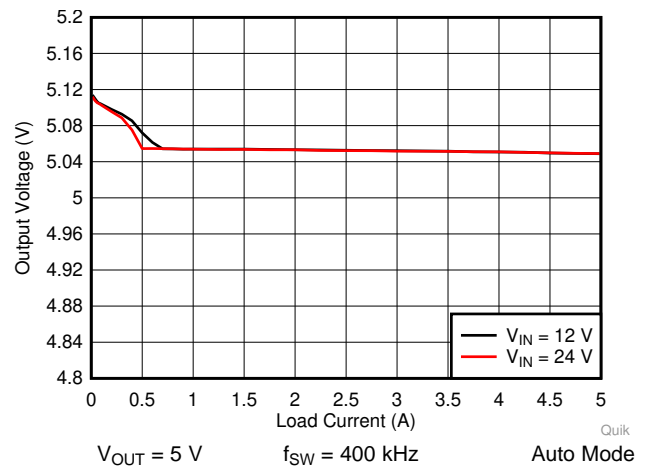
图 19. LM76005-Q1 Load and Line Regulation
