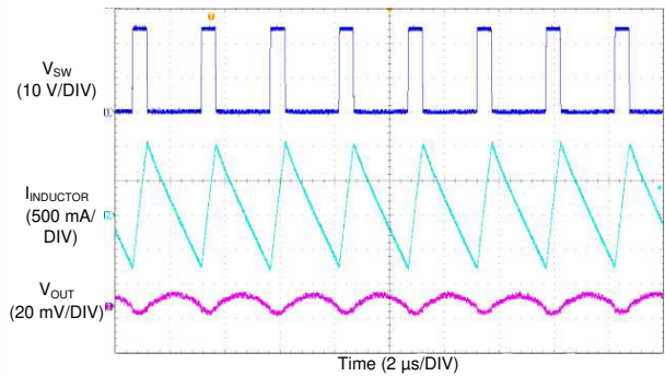
图 27. LM76005-Q1 Switching Waveform and Output Ripple
