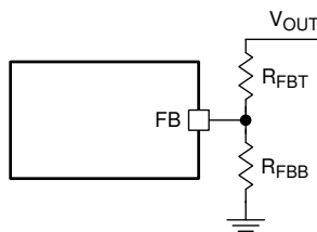
图 7. Output Voltage Setting
