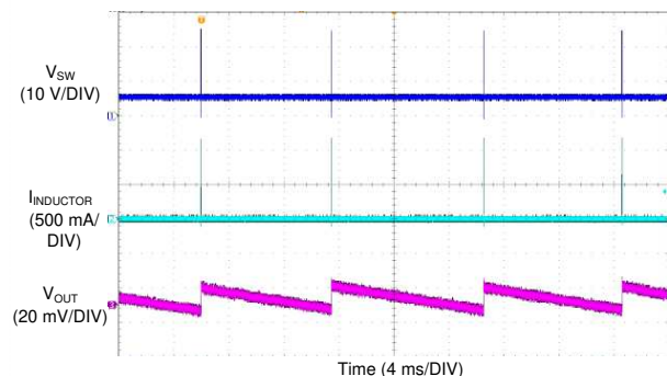
图 21. LM76005-Q1 Frequency Dropout
