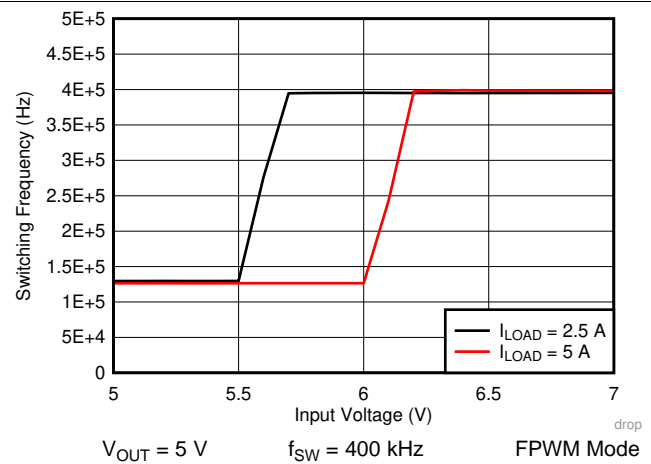
图 21. LM76005-Q1 Frequency Dropout
