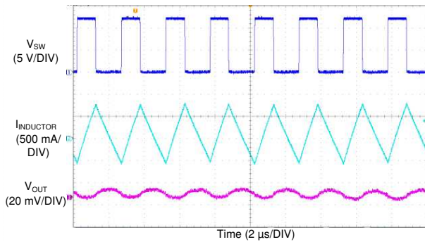
图 26. LM76005-Q1 Switching Waveform and Output Ripple
