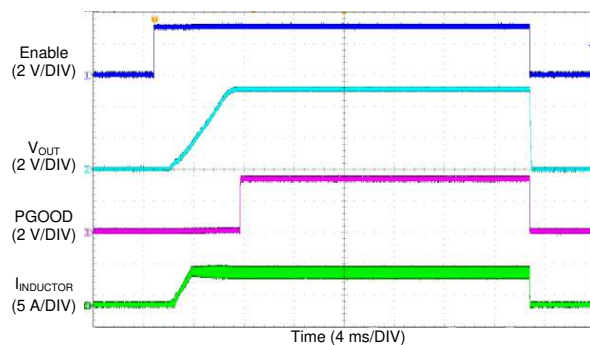
图 32. LM76005-Q1 Start-up Waveform
