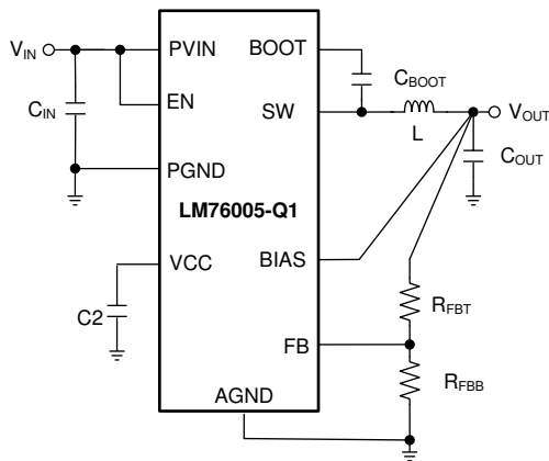
简化原理图
