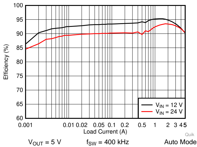
图 18. LM76005-Q1 Efficiency
