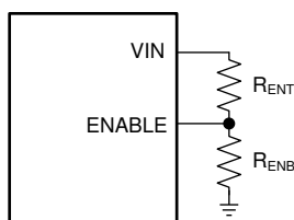
图 8. V_{IN} UVLO
