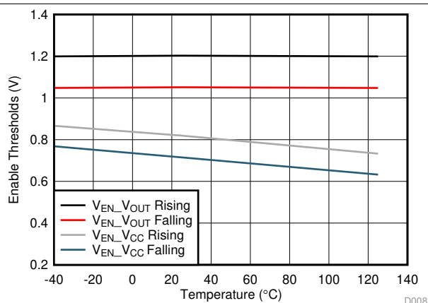
图 4. Enable Threshold
