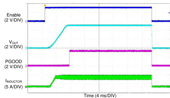
图 33. LM76005-Q1 Start-up Waveform
