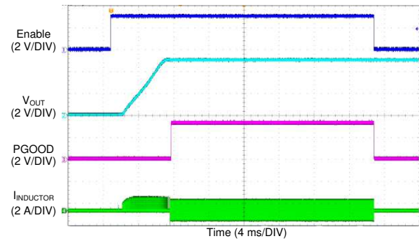
图 31. LM76005-Q1 Start-up Waveform
