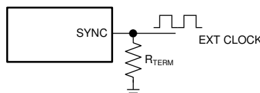
图 12. Frequency Synchronization
