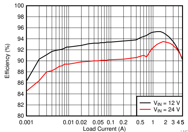
效率: V_{OUT} = 5V , f_{SW} = 400\text{kHz} , 自动模式
