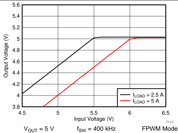
图 20. LM76005-Q1 Voltage Dropout
