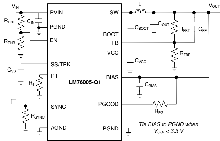
图 16. LM76005-Q1 Comprehensive Schematic
