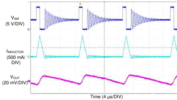
图 24. LM76005-Q1 Switching Waveform and Output Ripple
