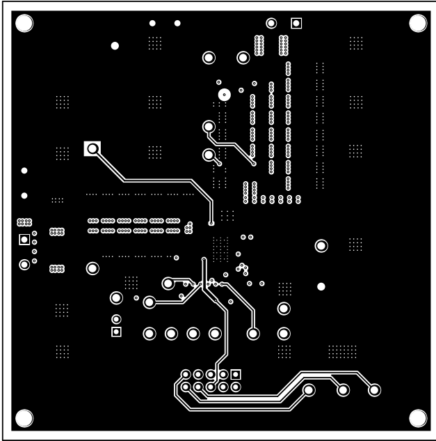
图 65. EVM Inner Layer 3
