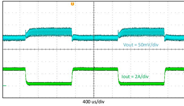
图 9-8. Transient Load Response, 0.3 to 2.7 A
