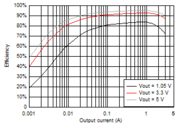
TPS563202S 效率
