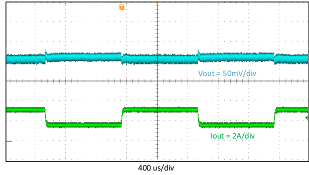
图 9-9. Transient Load Response, 1.5 to 3 A
