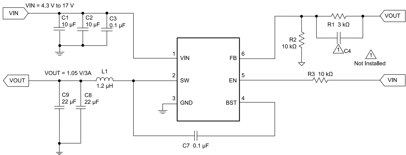
图 9-1. TPS563202S 1.05-V/3-A Reference Design
