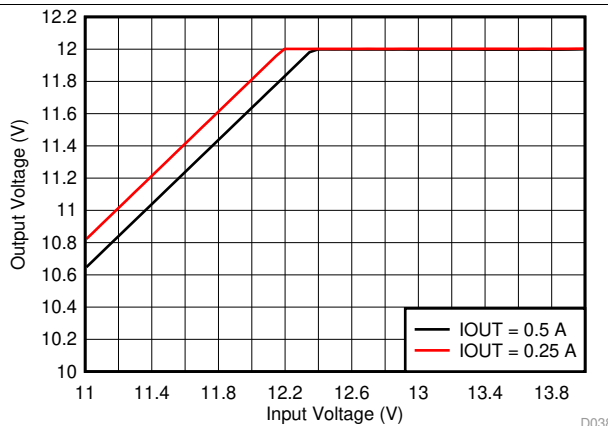
图 3. Dropout Voltage
