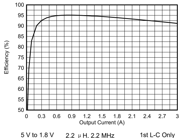
图 8-9. Efficiency vs Load Current
