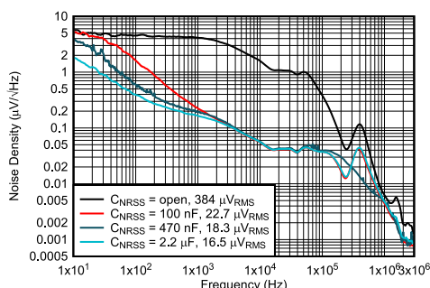
输出噪声与频率间的关系
