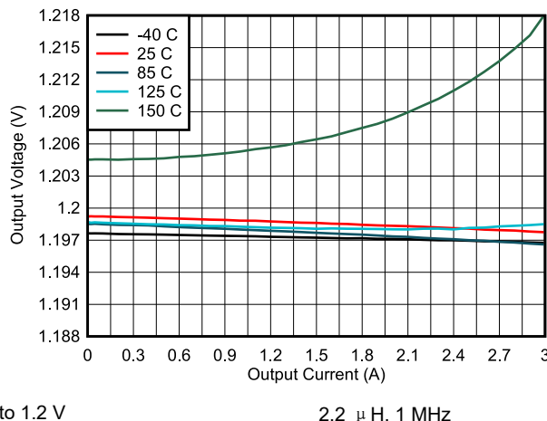
图 8-10. Output Voltage vs Load Current
