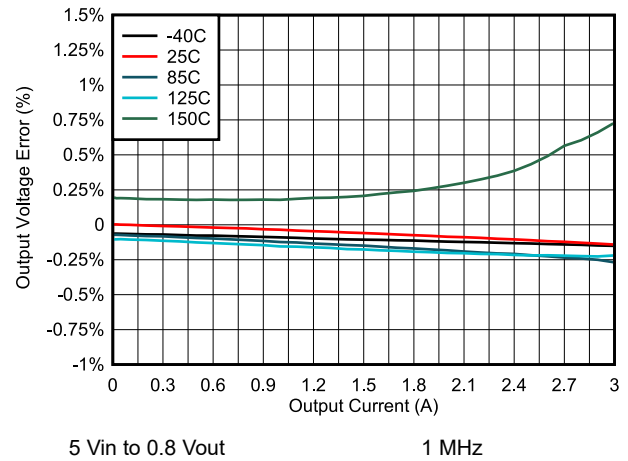
图 6-40. Output Voltage Error vs Load
