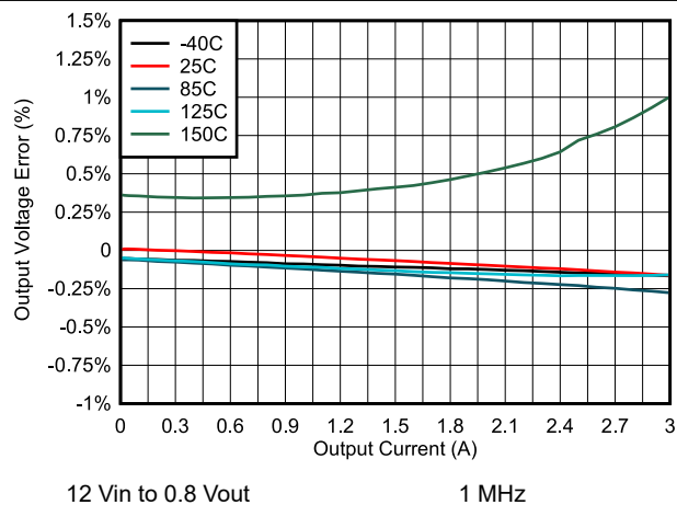
图 6-41. Output Voltage Error vs Load
