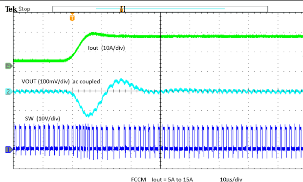
图 6-12. FCCM Mode Load Transient
