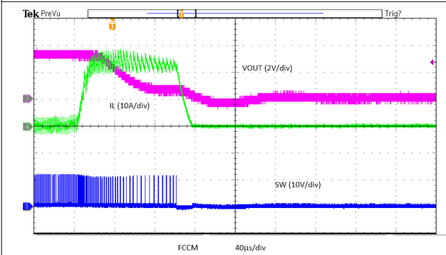
图 6-21. Overcurrent Protection
