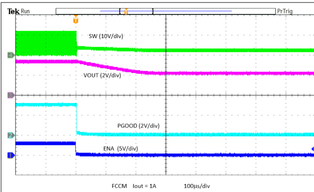
图 8-20. Prebias Power-Down
