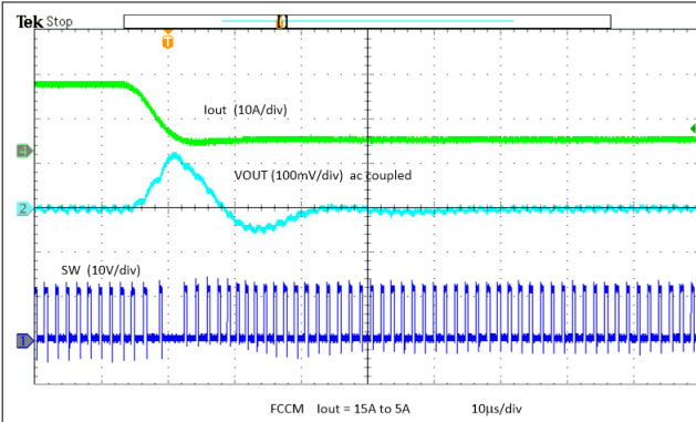
图 8-26. Unload Transient
