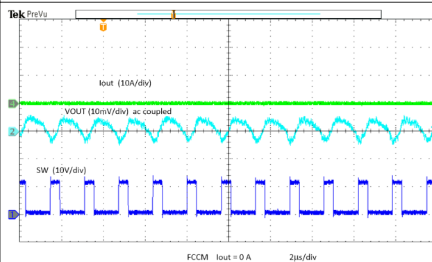
图 6-18. Vout Ripple, FCCM, No Load
