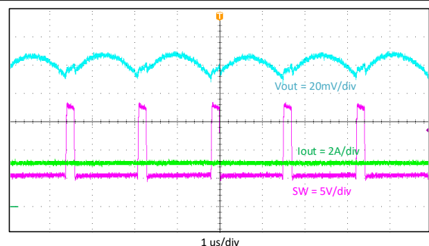
图 9-7. Output Voltage Ripple, I_{out} = 3\text{ A}
