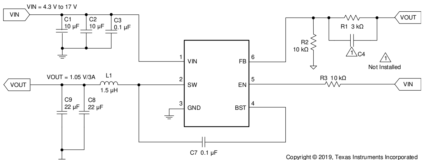
图 9-1. TPS563207 1.05-V/3-A Reference Design
