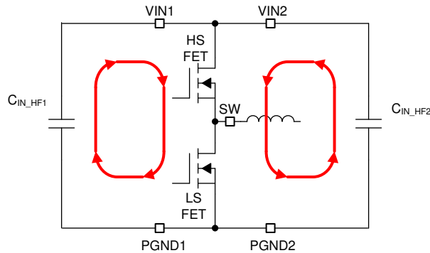
图 97. Input Current Loop
