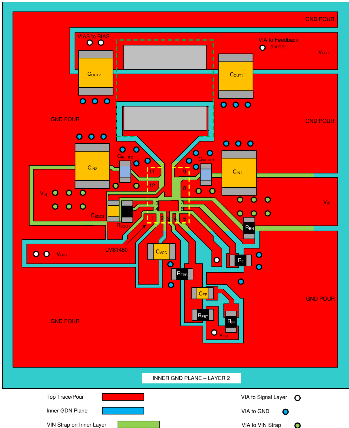
图 98. Layout Example
