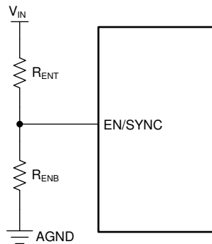
图 33. UVLO Using EN
