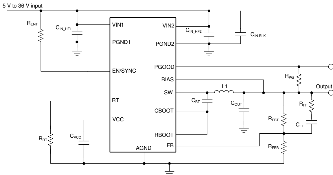
图 30. Example Application Circuit
