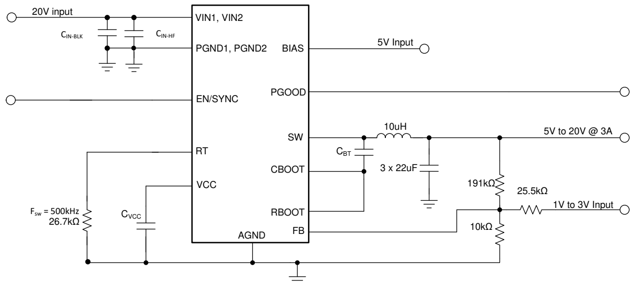
图 94. USB Type-C Power Supply
