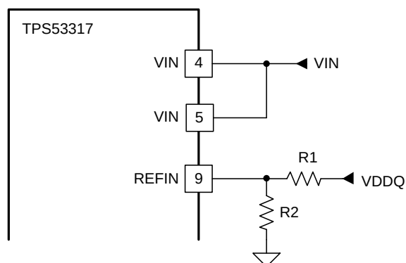
图 20. Tracking Configuration 2
