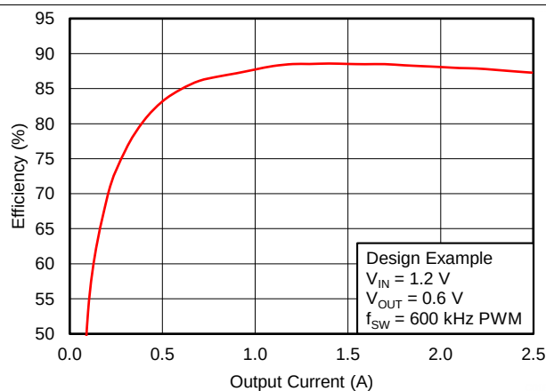
图 31. Efficiency
