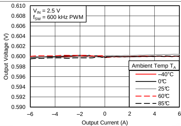
图 7. Load Regulation
