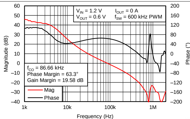
图 33. Bode Plot, No Load
