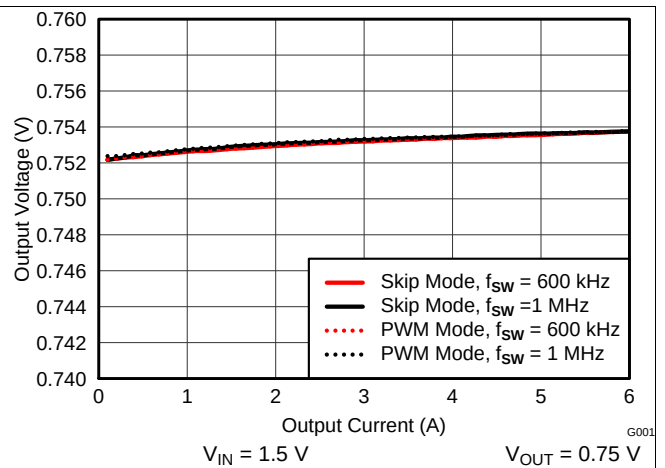
图 12. Load Regulation
