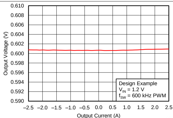
图 36. Load Regulation
