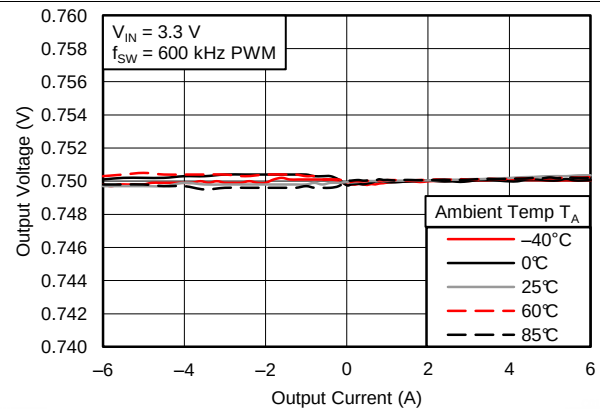
图 12. Load Regulation
