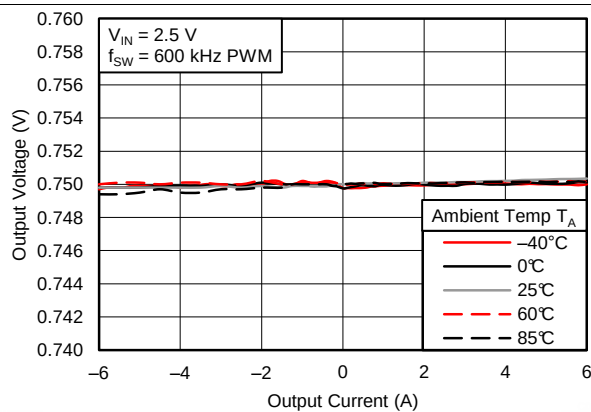
图 8. Load Regulation
