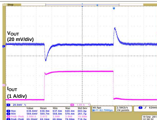
图 32. Load Transient
