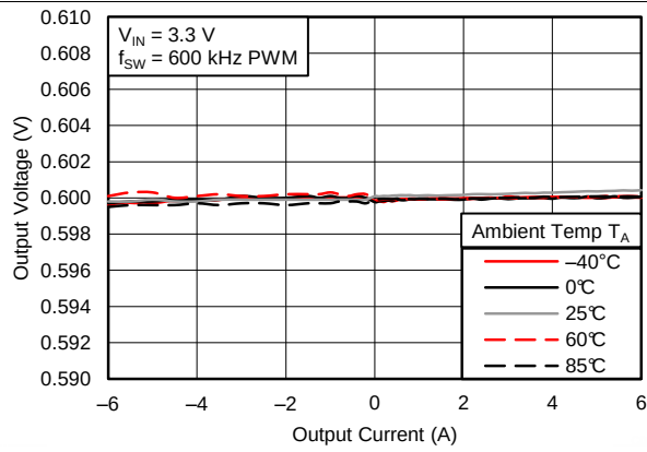
图 11. Load Regulation
