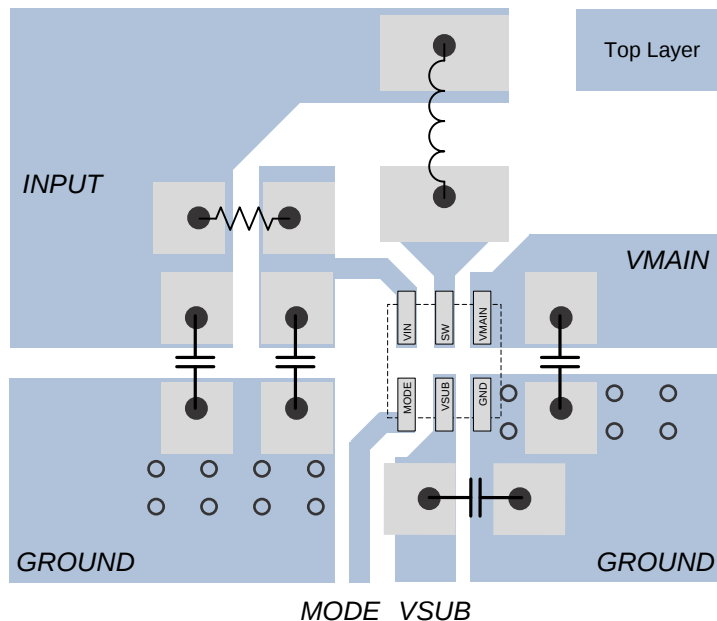
图 78. Layout
