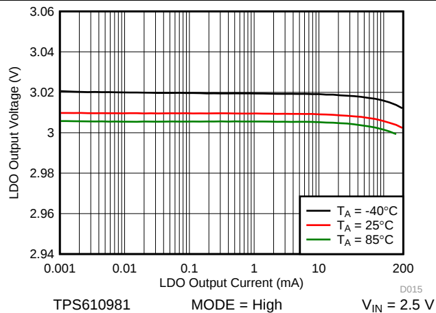
图 27. LDO Load Regulation
