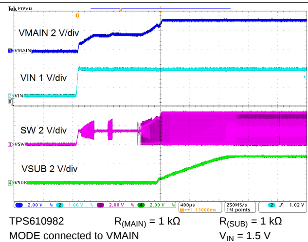
图 77. Startup
