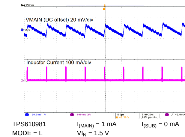
图 45. Switching Waveforms
