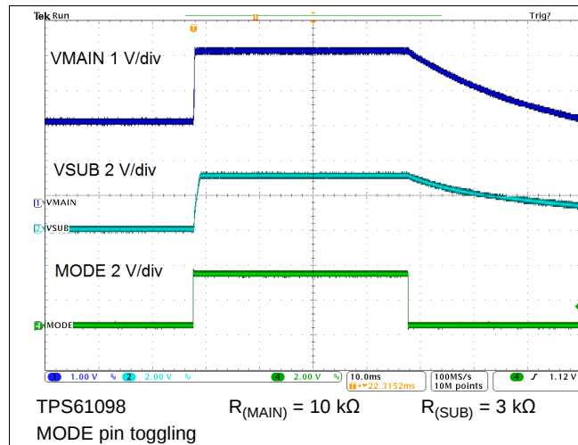
图 74. MODE Toggling
