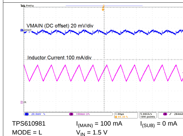
图 47. Switching Waveforms
