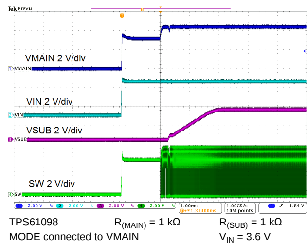
图 75. Startup
