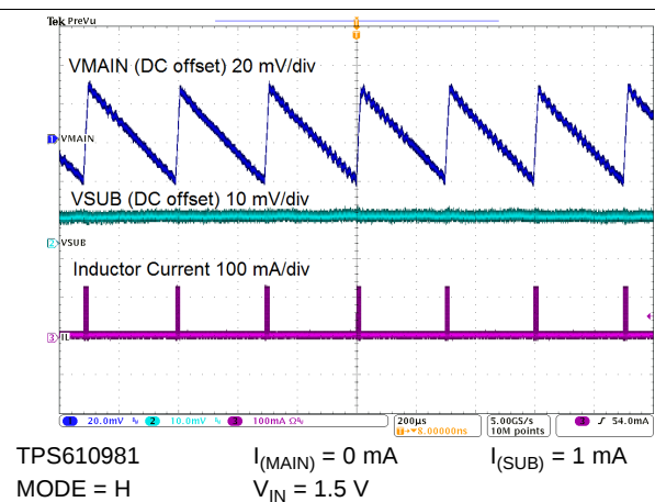
图 48. Switching Waveforms
