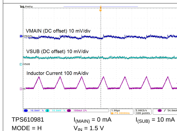
图 49. Switching Waveforms
