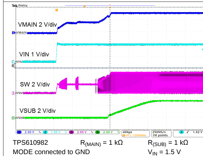
图 76. Startup
