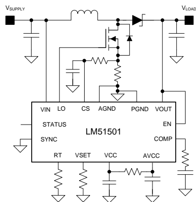
典型应用电路
