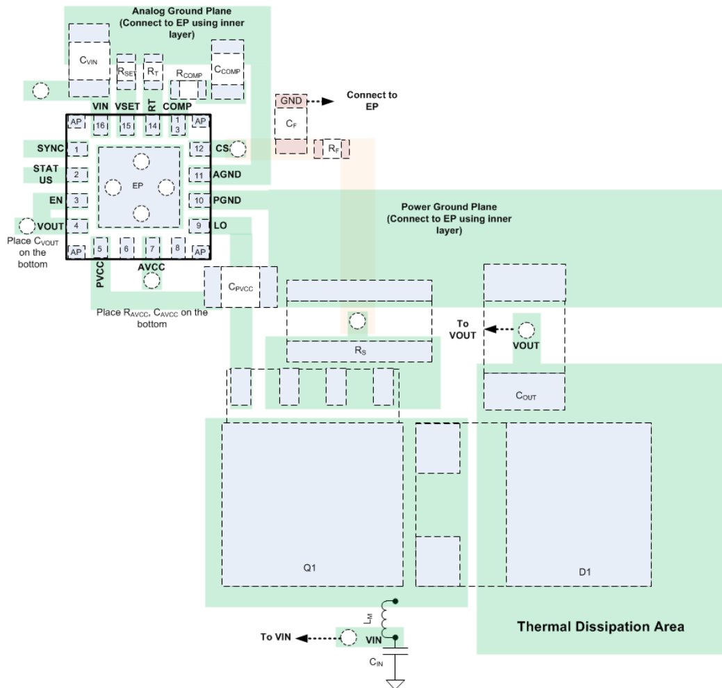
图 27. LM51501-Q1 PCB Layout Example
