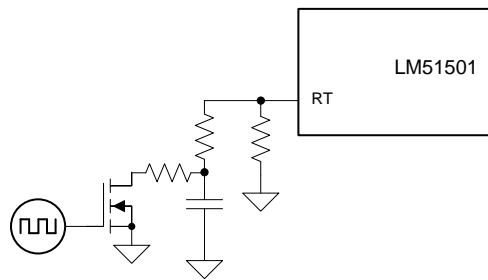
图 26. Dithering Using an External Clock
