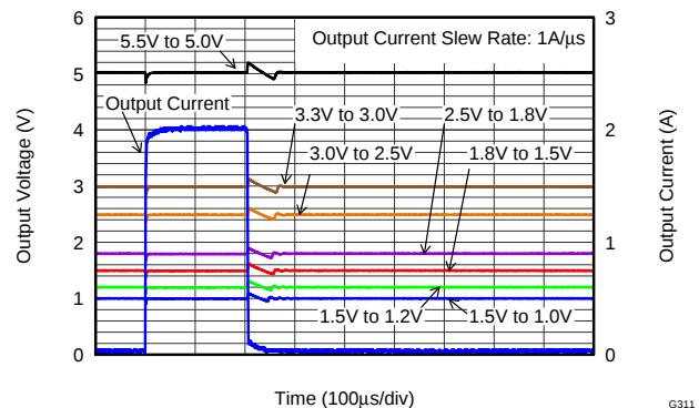
负载瞬态响应 (7 种不同输出)
