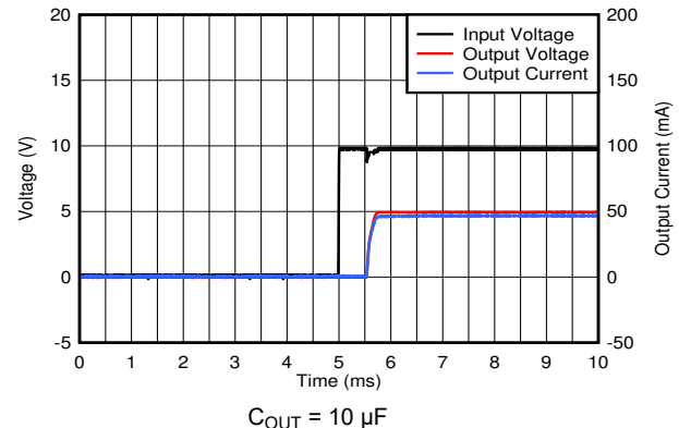
图 6-34. Startup Plot
