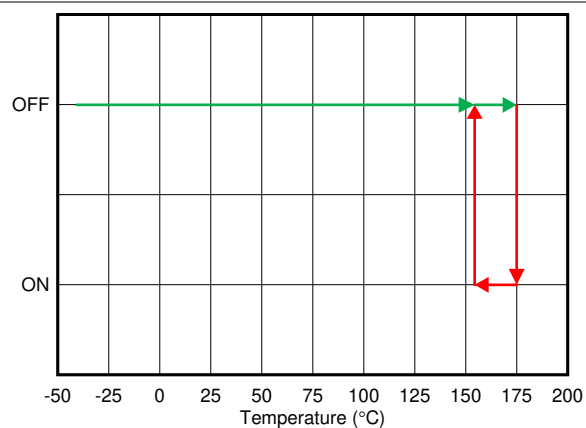
图 6-37. Thermal Shutdown
