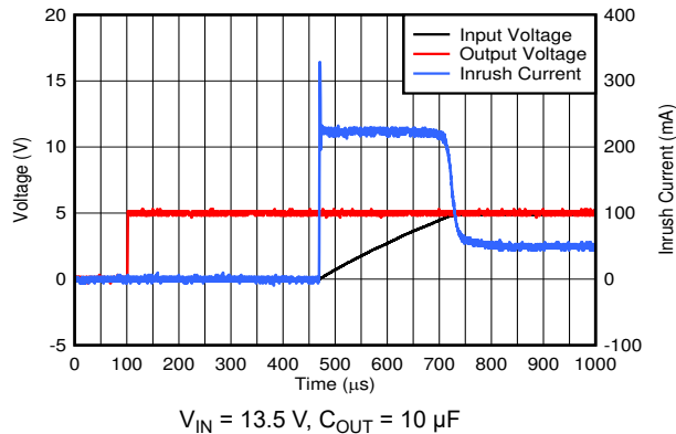
图 6-33. Startup Plot With EN
