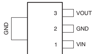
TLV1171xxDCY
