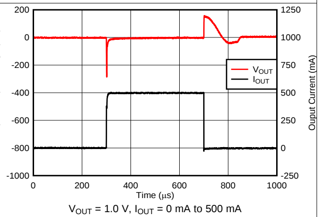
图 22. I_{OUT} Transient
