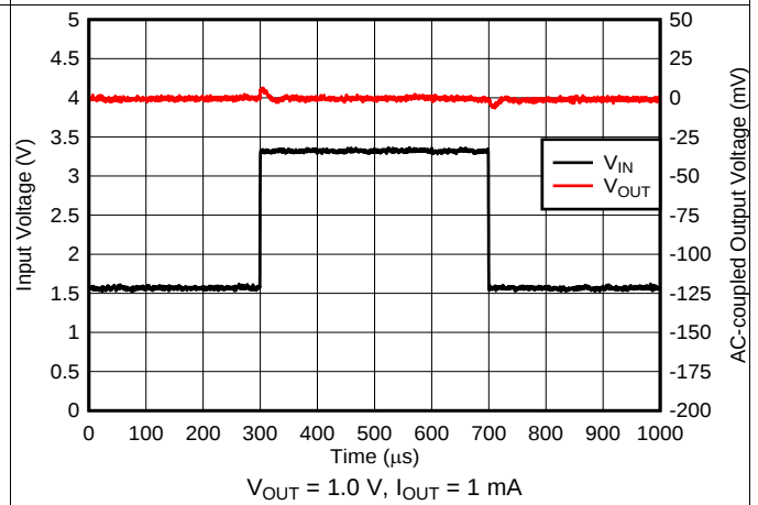
图 18. V_{IN} Transient
