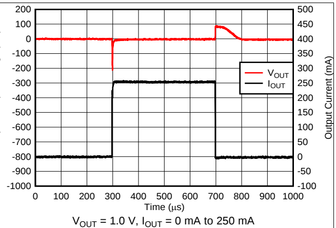
图 20. I_{OUT} Transient
