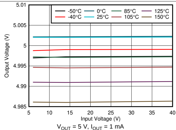
图 12. Output Voltage vs Input Voltage
