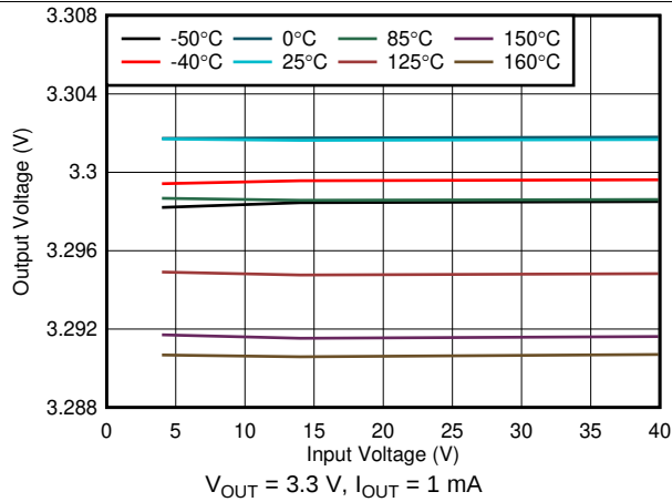
图 13. Output Voltage vs Input Voltage
