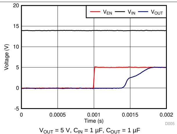
图 18. Startup With Enable
