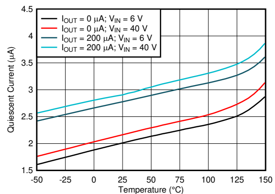
静态电流与环境温度间的关系 ( V_{OUT} = 3.3V )
