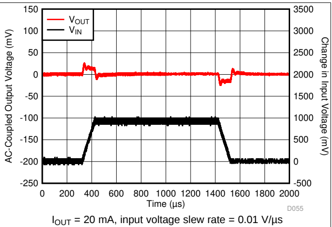
图 20. V_{IN} Transient
