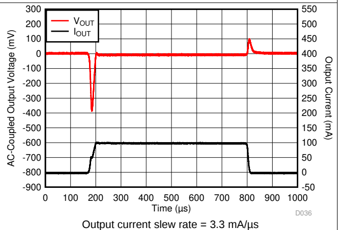
图 6. I_{OUT} Transient 0\text{ mA} to 100\text{ mA}
