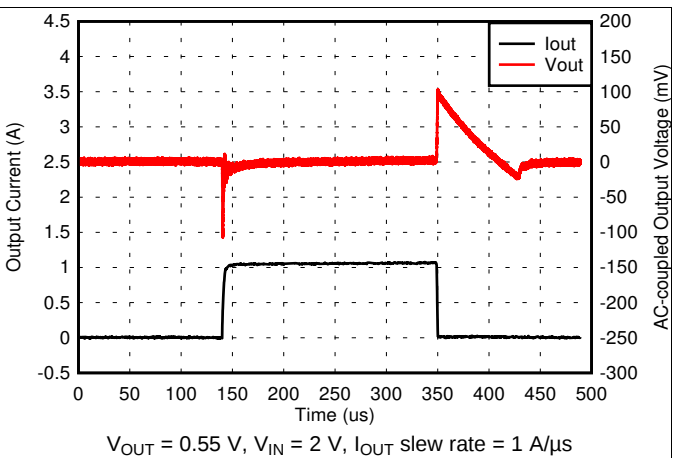
图 20. 1-mA to 1-A Load Transient (0.55 V)
