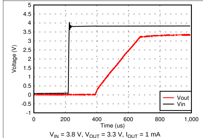
图 23. VIN Power-Up
