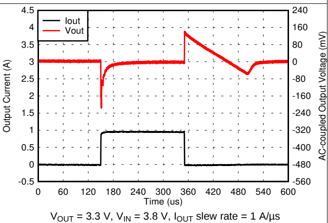
图 22. 1-mA to 1-A Load Transient (3.3 V)
