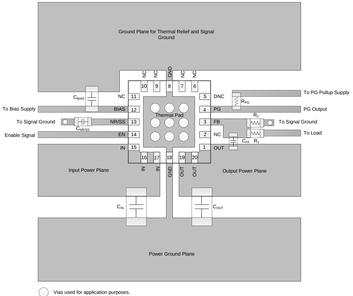
图 50. Example Layout
