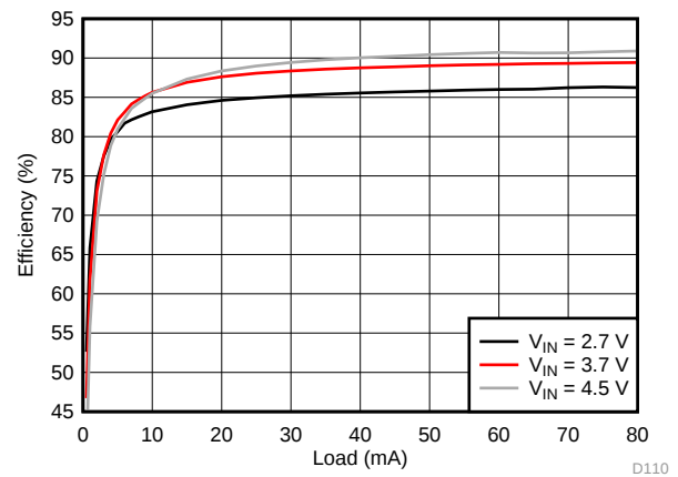
图 158. VPOS Efficiency
