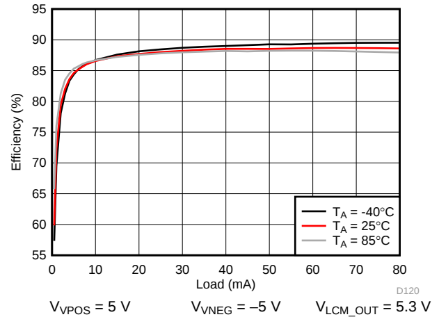
图 170. VPOS/VNEG Efficiency
