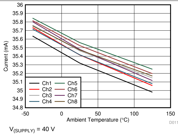
图 7. I_{(IOUTx)} Current vs Temperature
