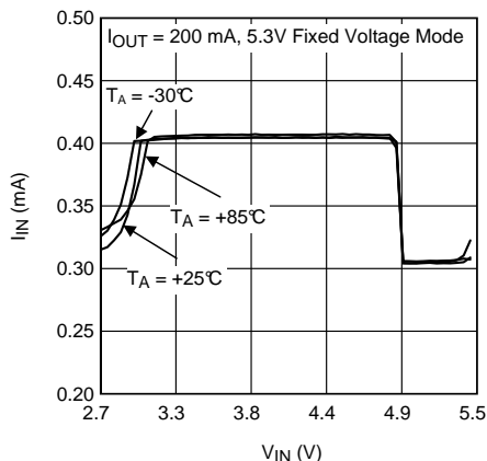
5.3-V Mode
