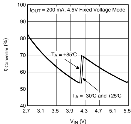
4.5-V Mode
