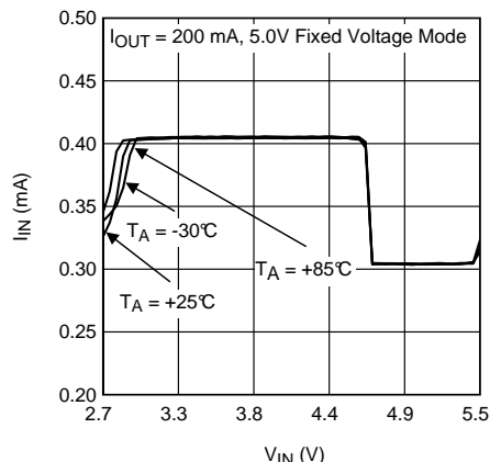
5-V Mode
