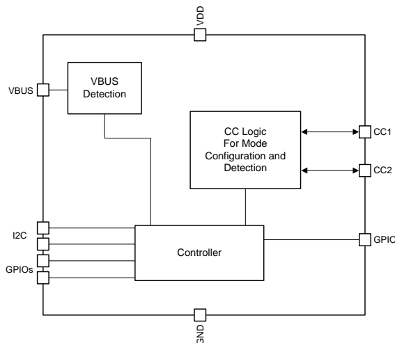
简化原理图
