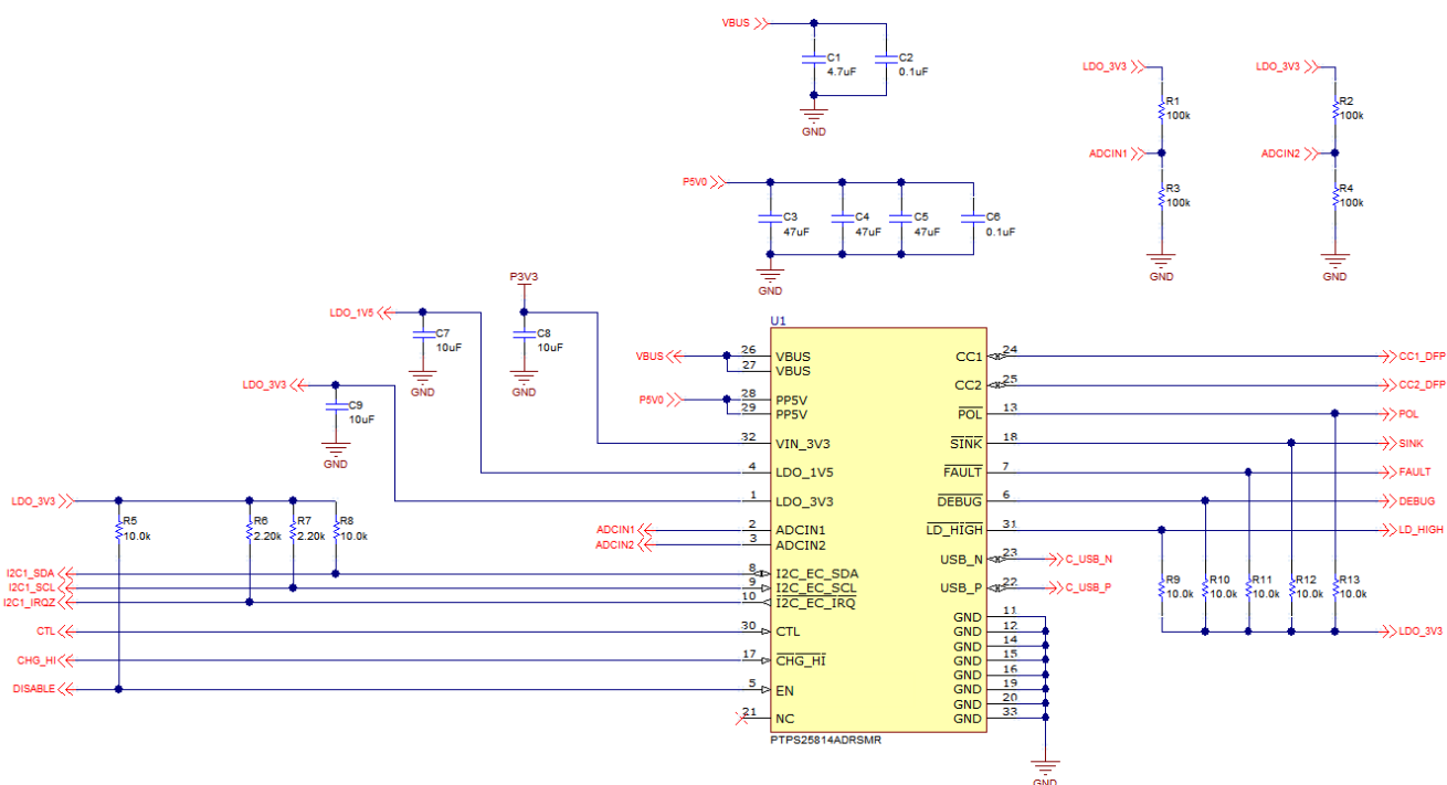
图 11-1. Example Schematic
