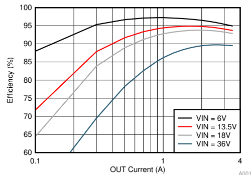
效率与输出电流间的关系 ( f_{\text{sw}} = 400\text{kHz} )
