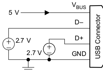
图 70. Divider 3 Mode
