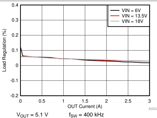
图 78. Load Regulation
