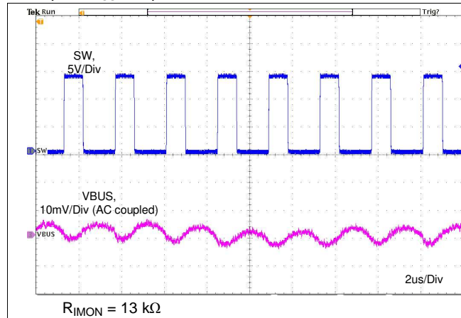
图 86. 100-mA Output Ripple
