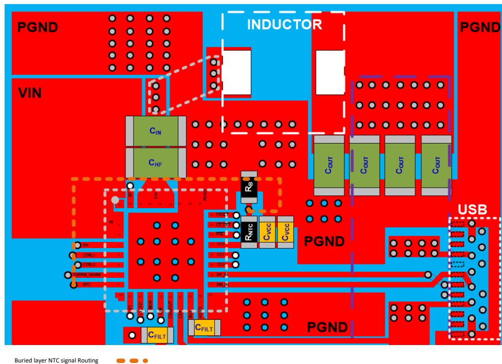
图 68. NTC Placement Example
