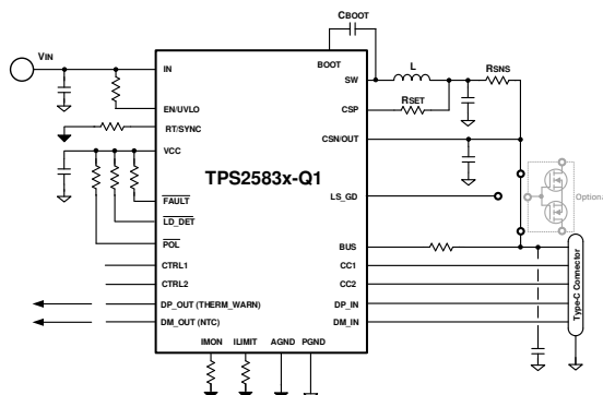
TPS2583x-Q1 简化原理图
