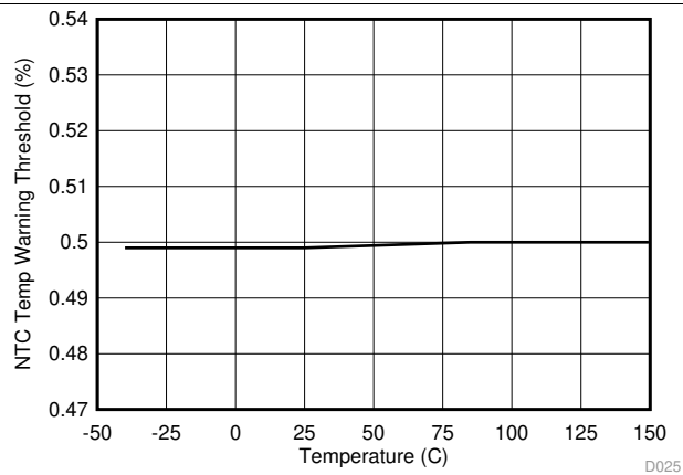
图 27. NTC Temperature Warning Threshold (TPS25833-Q1)
