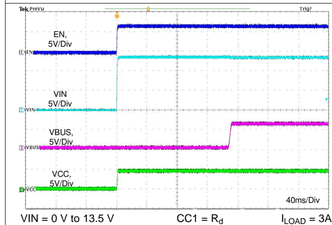
图 88. Startup Relate to VIN
