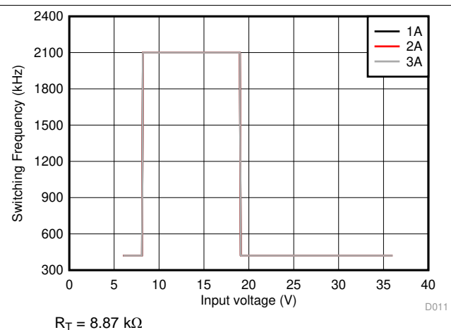
图 12. Switching Frequency vs VIN Voltage
