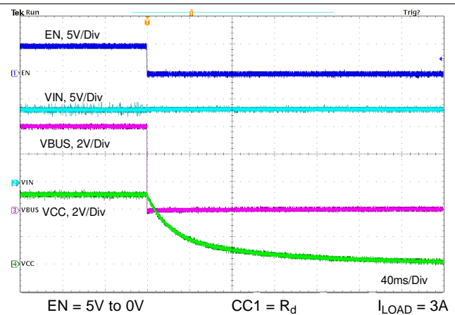
图 91. Shutdown Relate to EN
