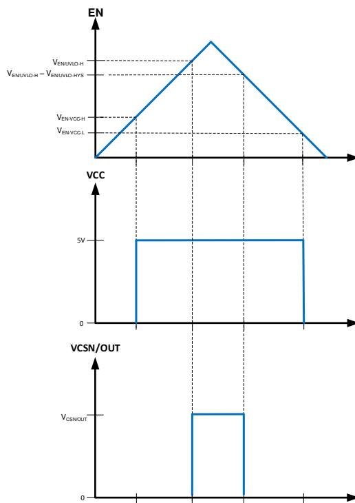
图 39. Precision Enable Behavior
