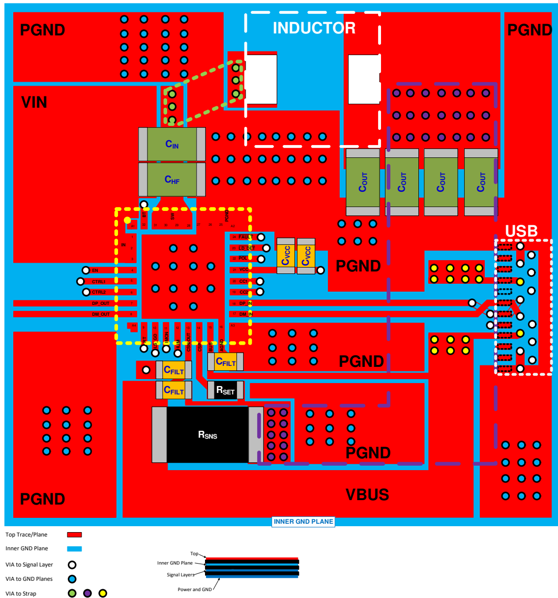
图 105. TPS2583x-Q1 Layout
