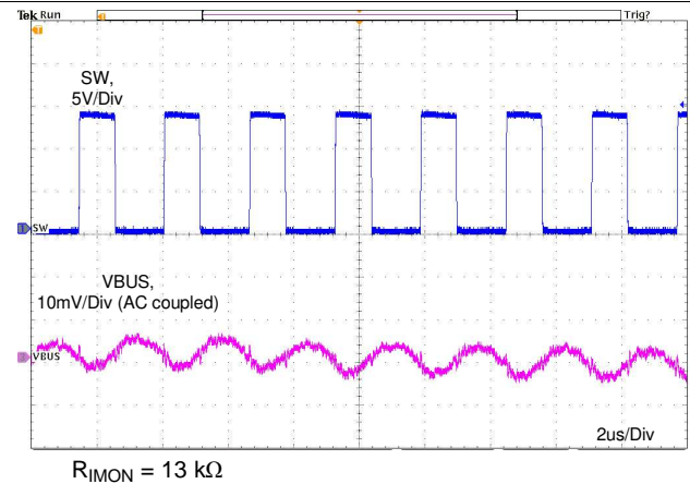
图 85. 3.5-A Output Ripple
