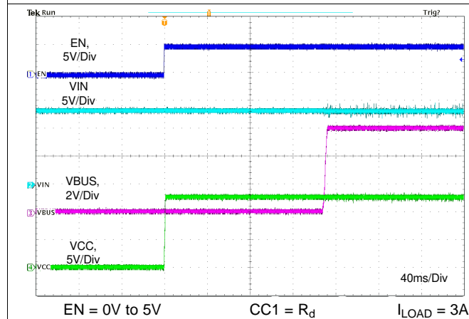
图 90. Startup Relate to EN
