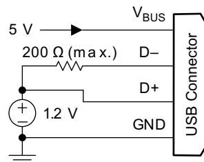
图 71. 1.2-V Mode
