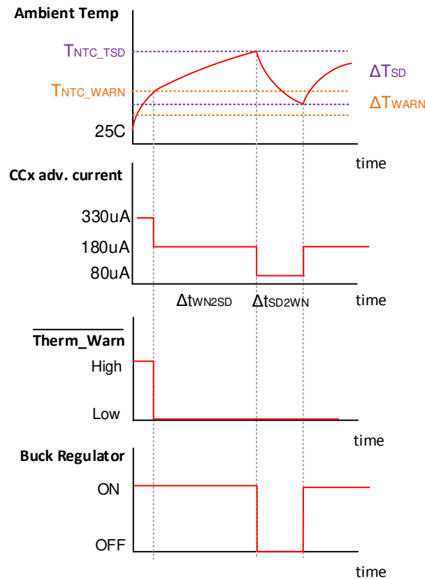
图 66. TPS25833-Q1 Behavior when Trigger NTC Threshold
