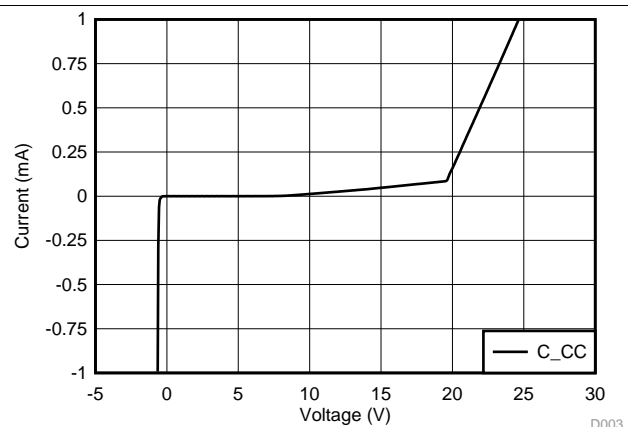
图 24. C_CC IV Curve
