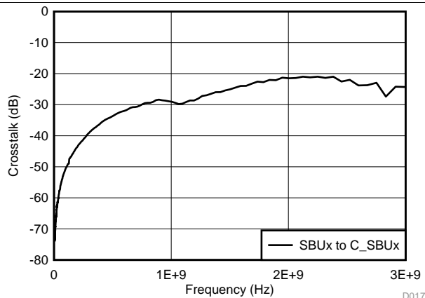
图 2. SBU Crosstalk
