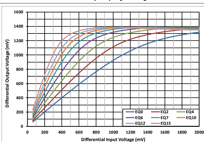
图 2. USB RX (DFP) EQ Settings Curves
