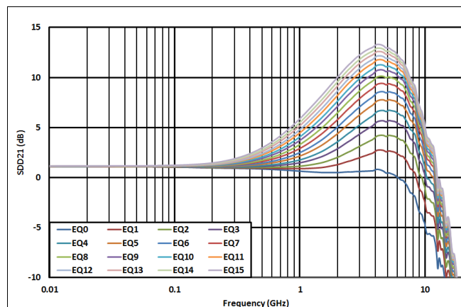
图 1. DisplayPort EQ Settings Curves
