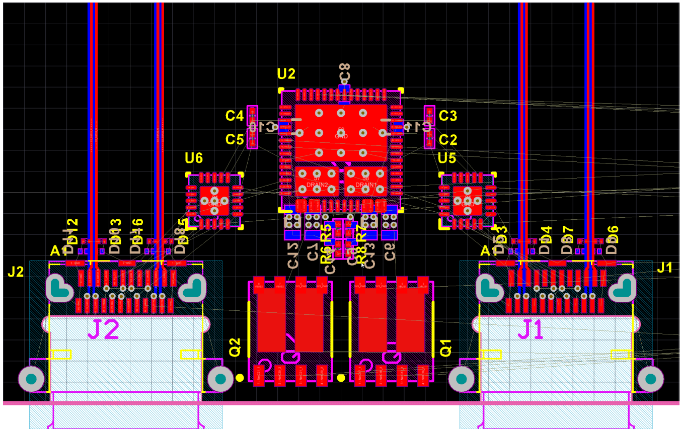
图 57. Protection Placement
