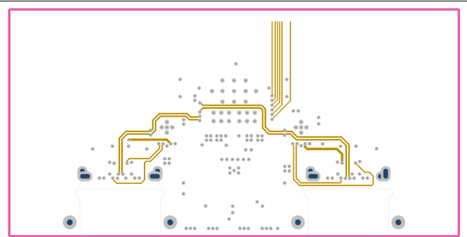
图 67. High Speed Layer
