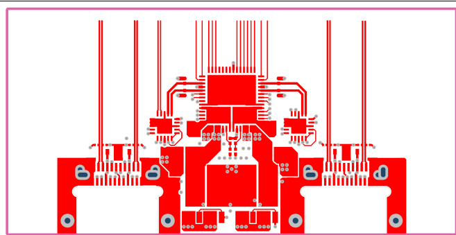
图 66. SSTXR1 Layer
