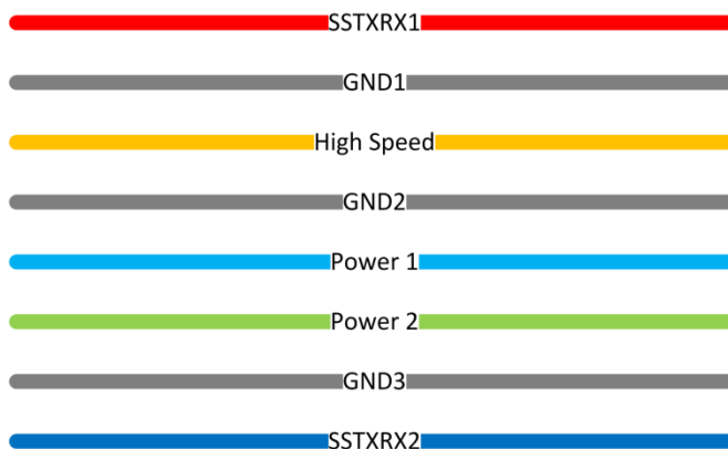
图 47. 8 Layer Board Stack Up
