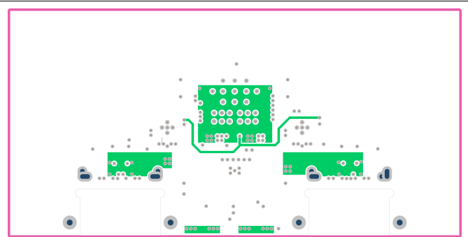
图 69. Power 2 Layer
