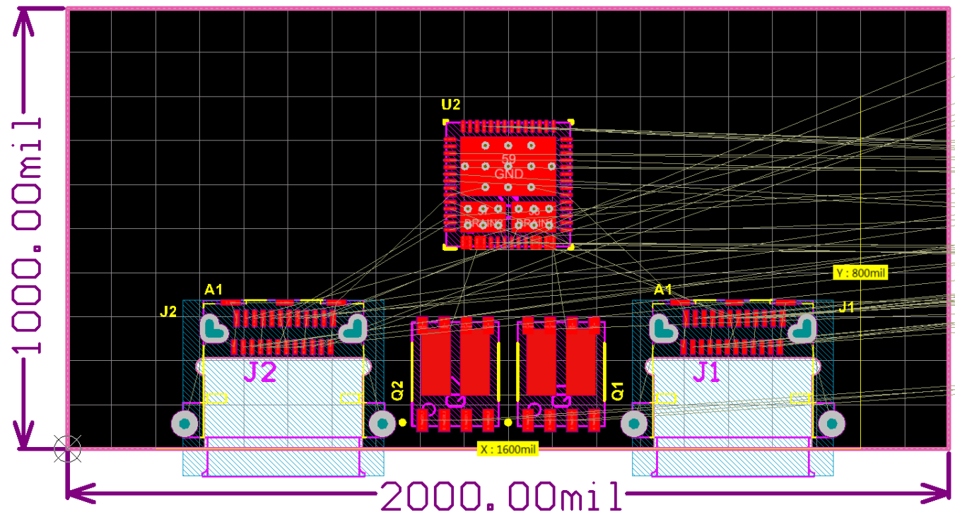
图 49. High Level Placement
