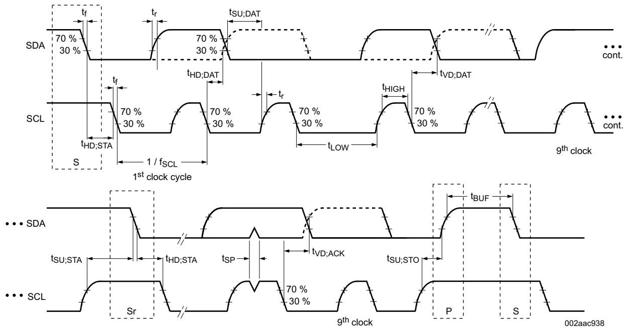
图 3. I 2 C Slave Interface Timing
