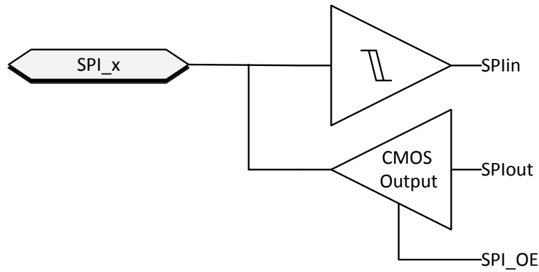
图 25. SPI buffer
