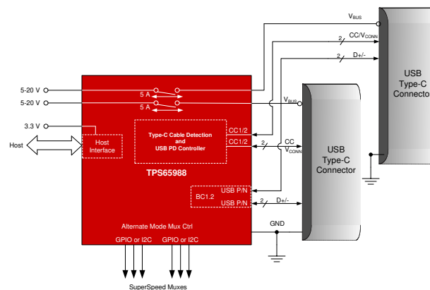
简化原理图
