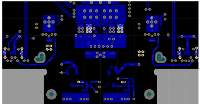
图 65. VBUS Routing Bottom Layer
