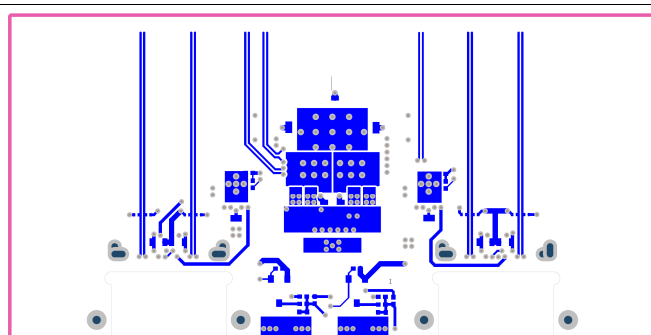
图 70. SSTXRX2 Layer
