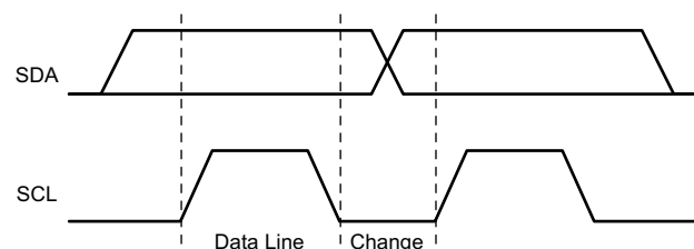
图 28. I 2 C Bit Transfer
