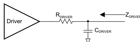
图 11. ZDRIVER Circuit
