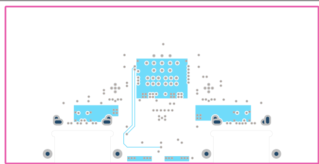
图 68. Power 1 Layer
