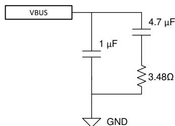
图 37. VBUS Snubber
