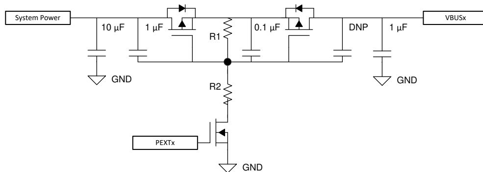
图 35. Simple Sink Power Path
