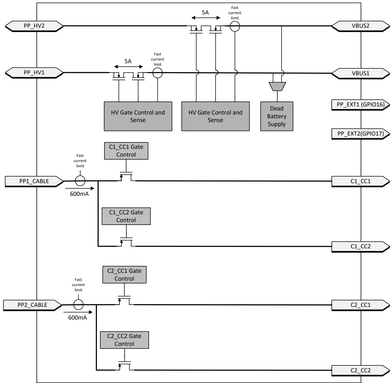
图 14. Port Power Switches
