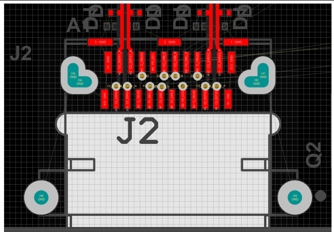
图 51. Type-C Connector SSTXRX Top Layer
