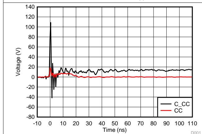
图 15. CC Short-to-V BUS 20 V
