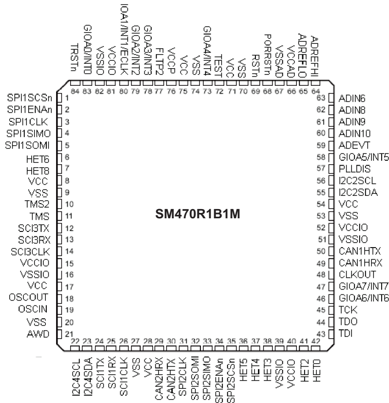
图 1. SM470R1B1M 84 引脚 CQFP-HFQ/HKP (顶视图)
