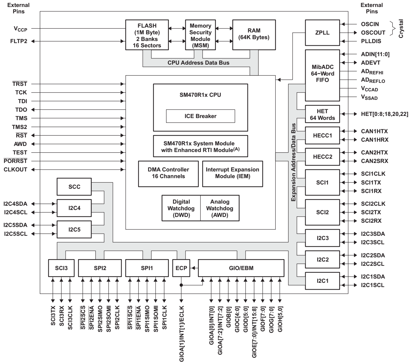
功能框图
