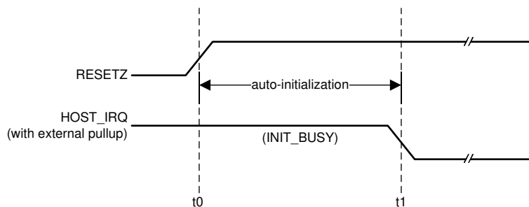
图 7-4. HOST_IRQ Timing
