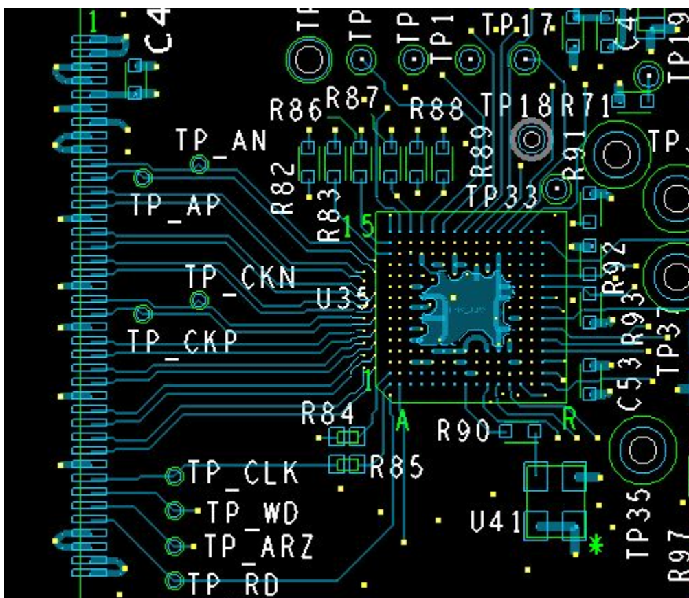
图 10-3. Layout Recommendation
